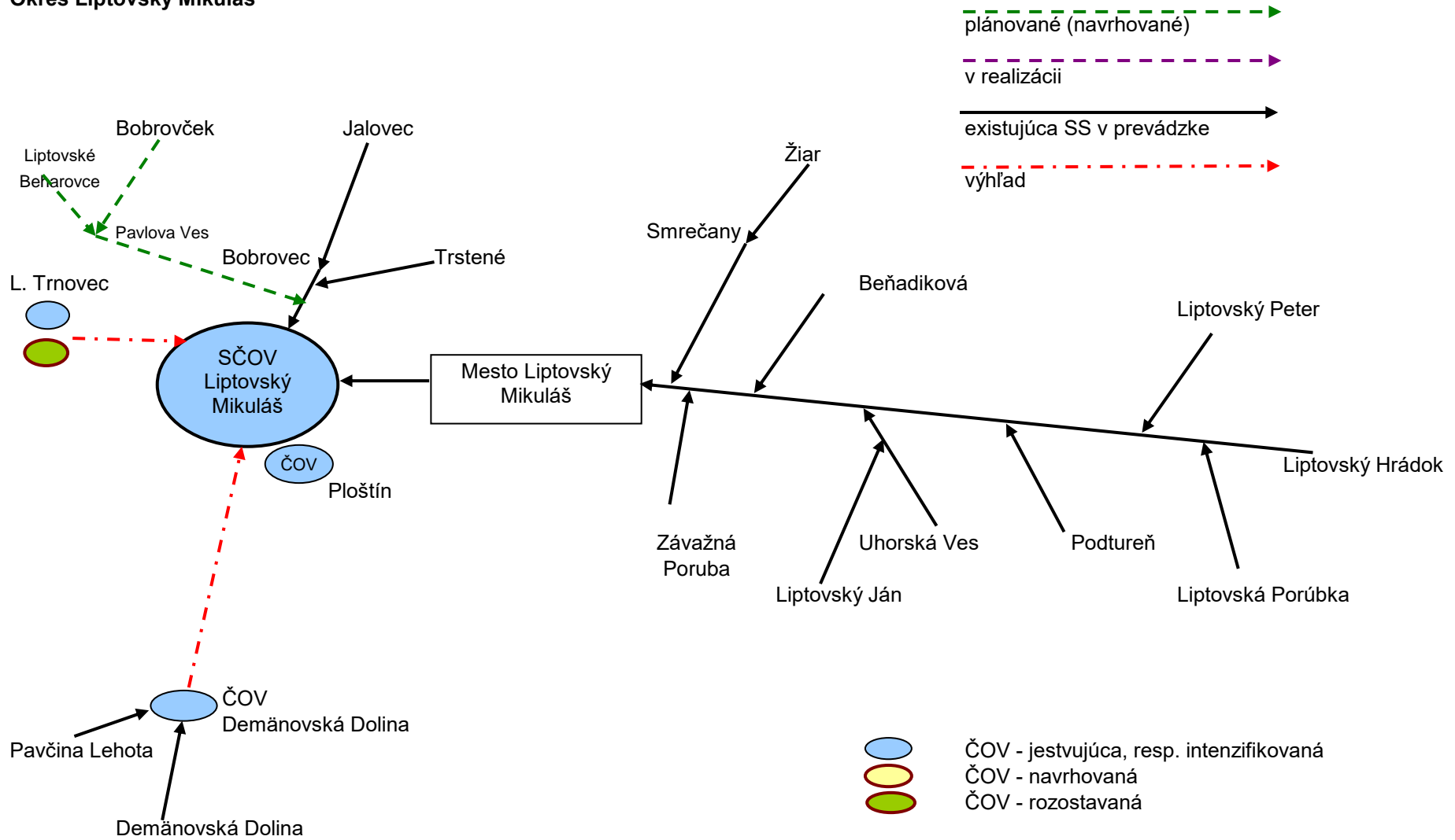
Schéma č. 1 - Schéma odvádzania a čistenia odpadových vôd Okres Liptovský Mikuláš
