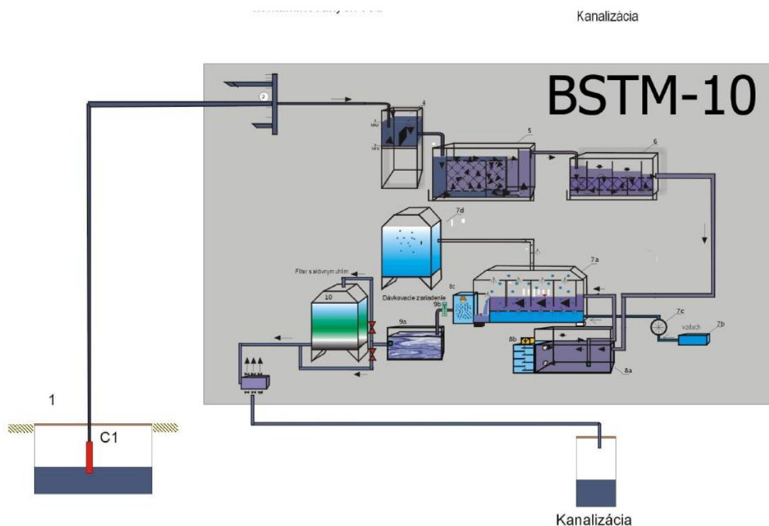
Obrázok č.1: Schéma funkcie mobilnej sanačnej linky BSTM-10 (Vid' Príloha č.2a)
