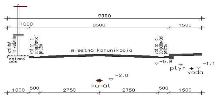
VZOROVÝ PRIEČNÝ REZ MIESTNOU KOMUNIKÁCIOU
