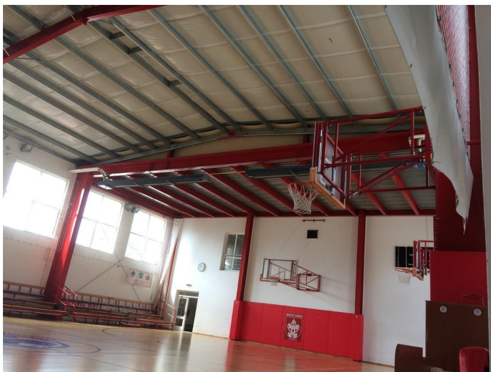
Obrázok 54: Interiér športovej haly Sokolovňa – vykurovanie infražiaľmi, reflektorové osvetlenie
