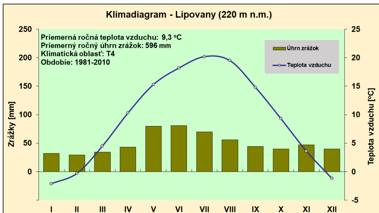
Obr.14 Klimadiagram obce Lipovany - súčasné klimatické podmienky (1981-2010)
