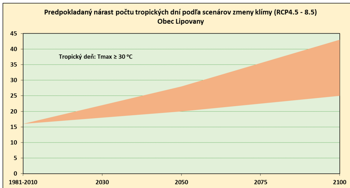
Obr.15 Predpokladaný nárast počtu tropických dní v obci Lipovany podľa RCP scenárov
