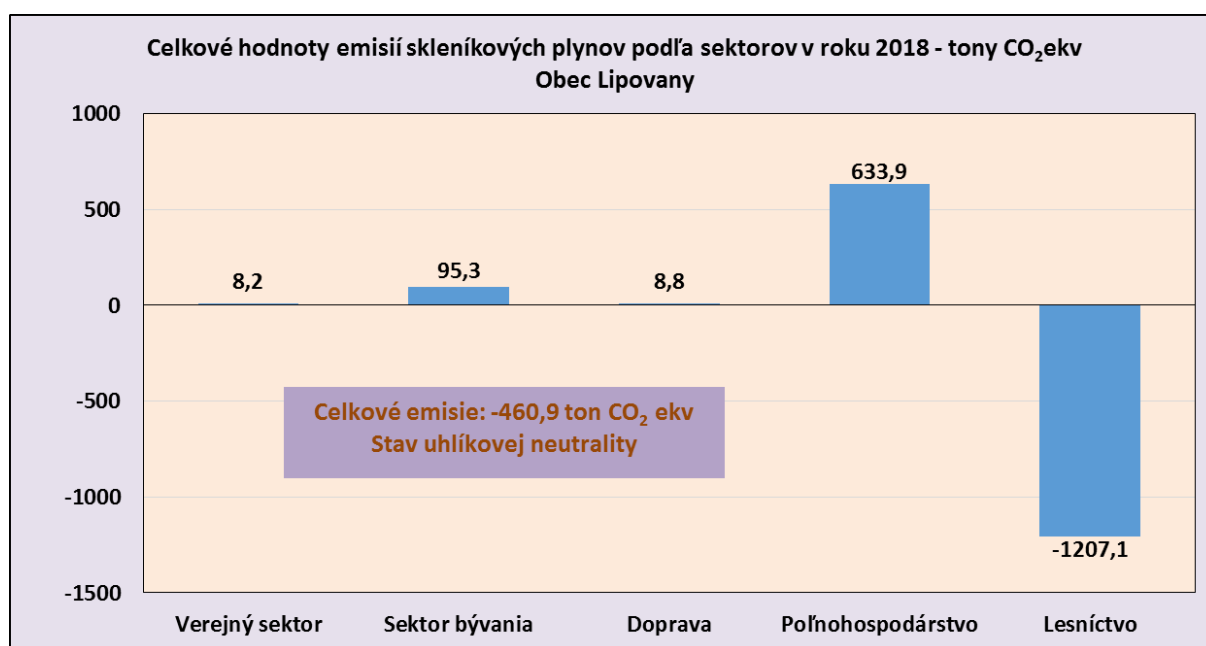
Obr.6 Celkové emisie skleníkových plynov v tonách CO 2 ekv za rok 2019 – obec Lipovany
