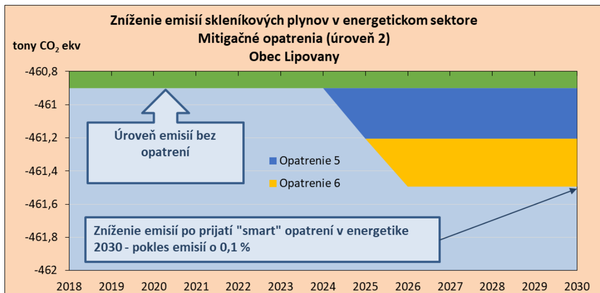
Obr.10 Zníženie emisií skleníkových plynov na báze prijatých mitigačných opatrení – obec Lipovany
