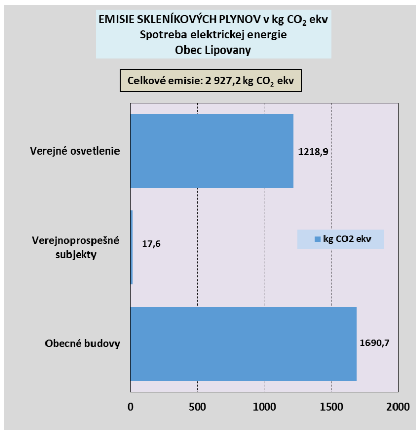
Obr.2 Emisie oxidu uhličitého (v kg CO 2 ekv) zo spotreby elektrickej energie pre obecné budovy – obec Lipovany
