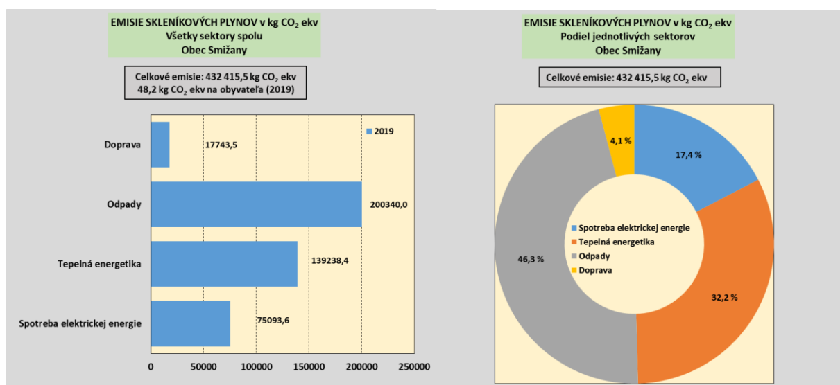
Obr.4 Podiel jednotlivých sektorov na celkových emisiách skleníkových plynov – verejný sektor obec Smižany
