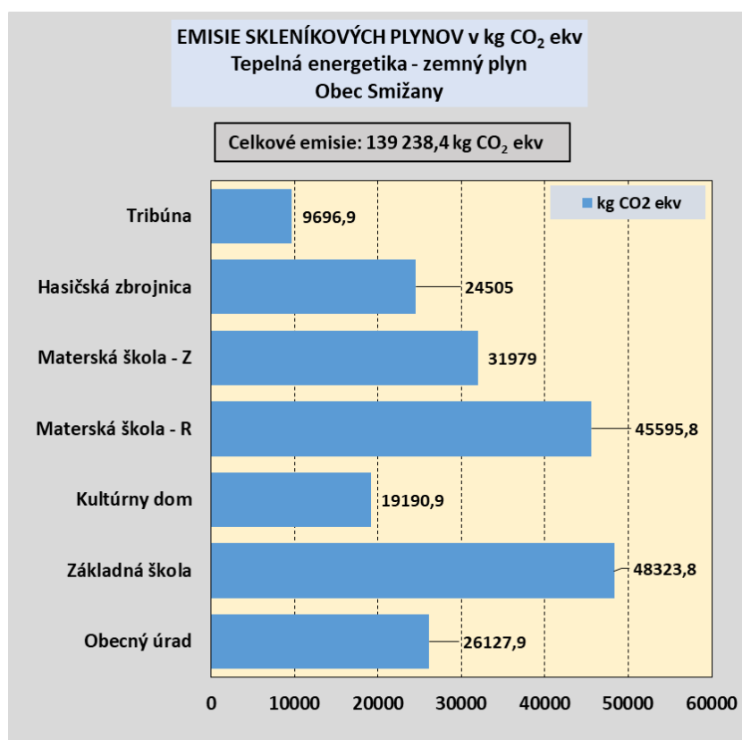
Obr.3 Emisie oxidu uhličitého (v kg CO 2 ekv) z tepelnej energetiky – obec Smižany
