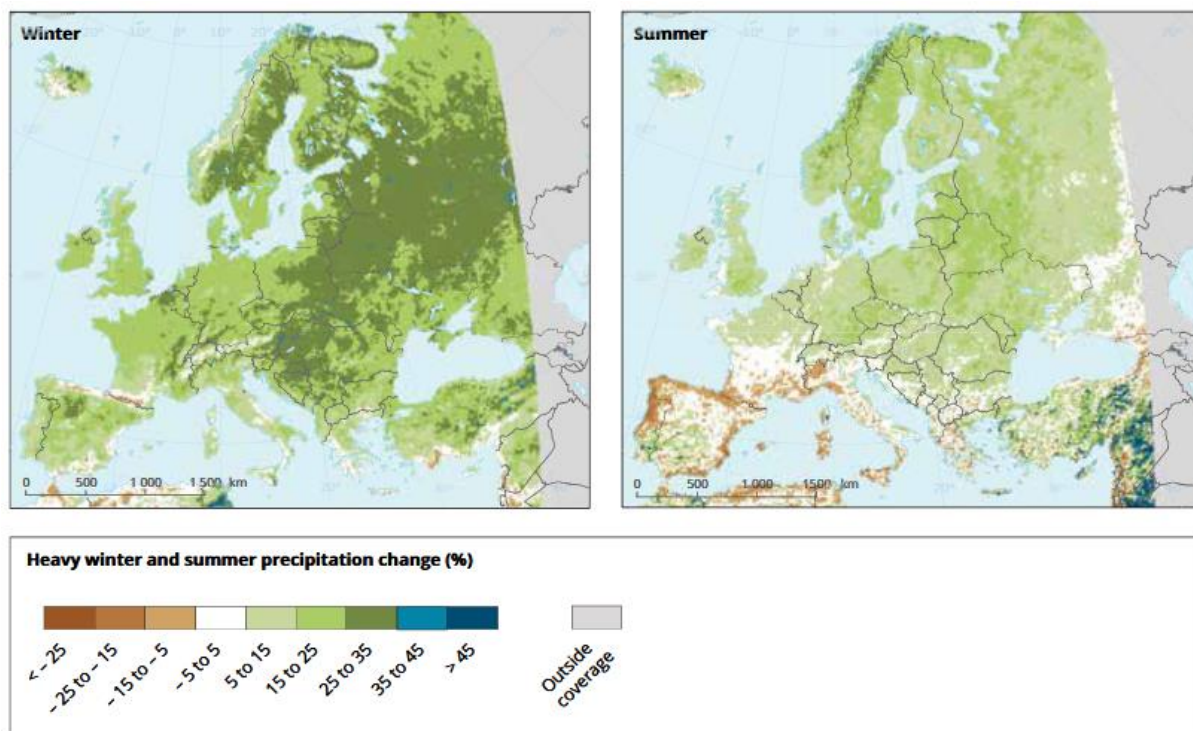
Obr.12 Predpokladané zmeny intenzívnych letných a zimných zrážok v Európe Zdroj: EURO-CORDEX (Jacob et al., 2014) ex EEA Report No 1/2017
