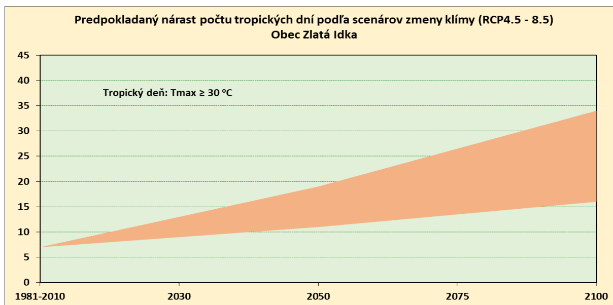
Obr.16 Predpokladaný nárast počtu tropických dní v obci Zlatá Idka podľa RCP scenárov
