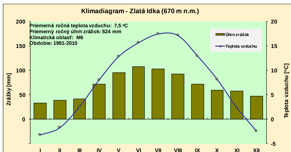
Obr.15 Klimadiagram obce Zlatá Idka - súčasné klimatické podmienky (1981-2010)
