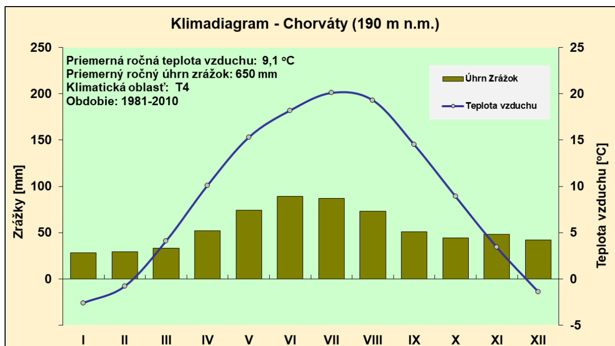
Obr.15 Klimadiagram obce Chorváty - súčasné klimatické podmienky (1981-2010)
