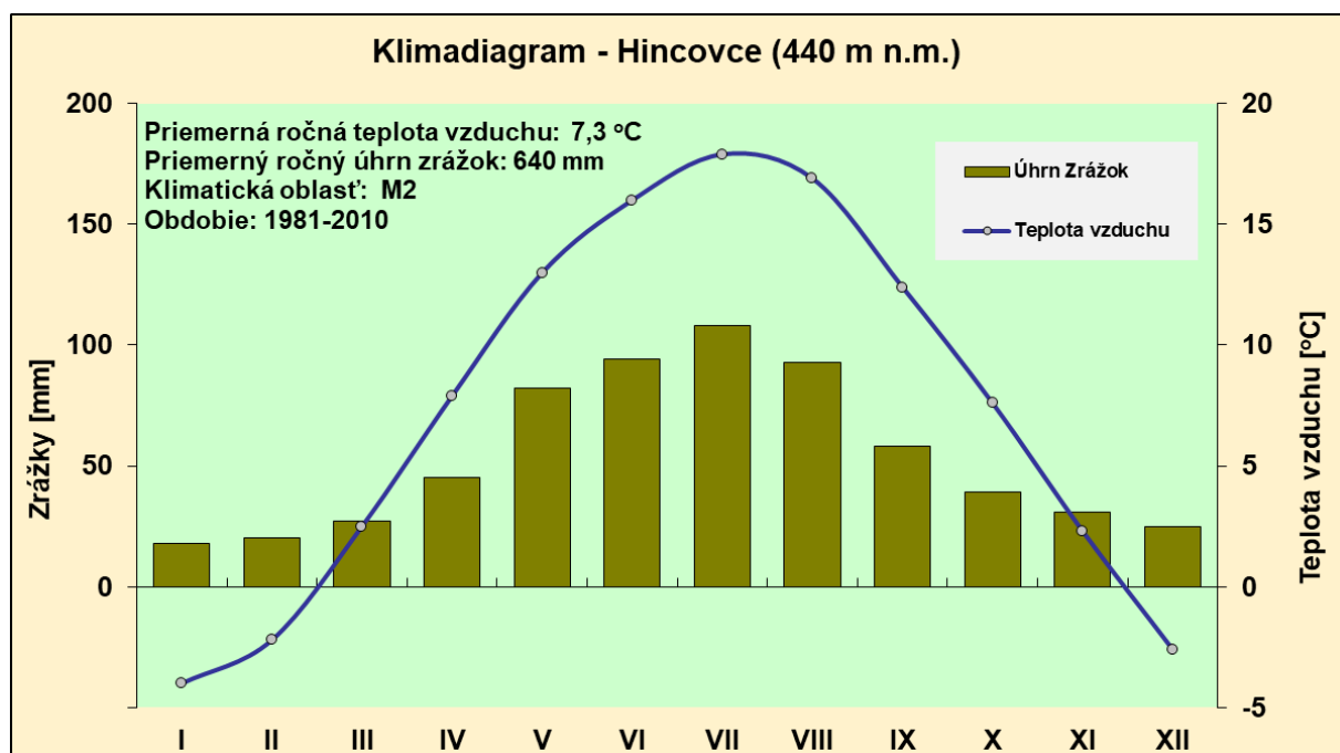
Obr.15 Klimadiagram obce Hincovce - súčasné klimatické podmienky (1981-2010)
