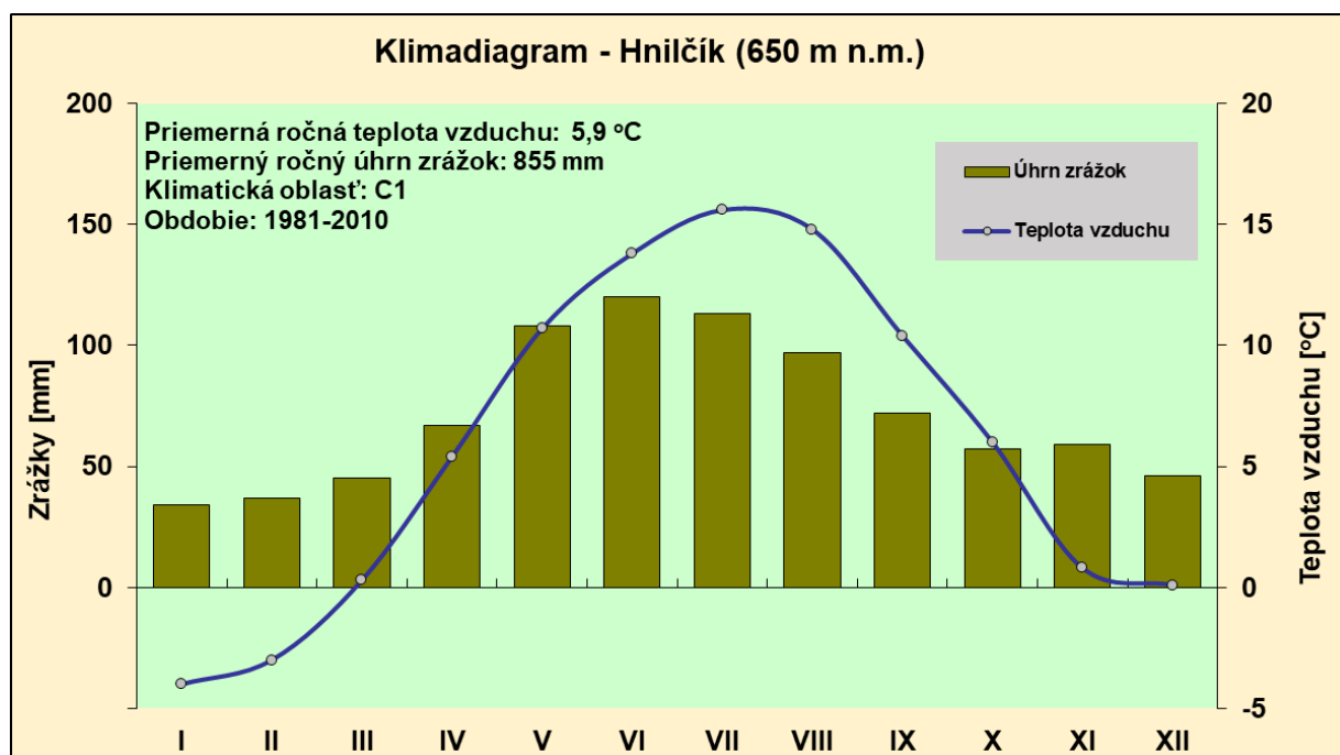
Obr.14 Klimadiagram obce Hnilčík - súčasné klimatické podmienky (1981-2010)
