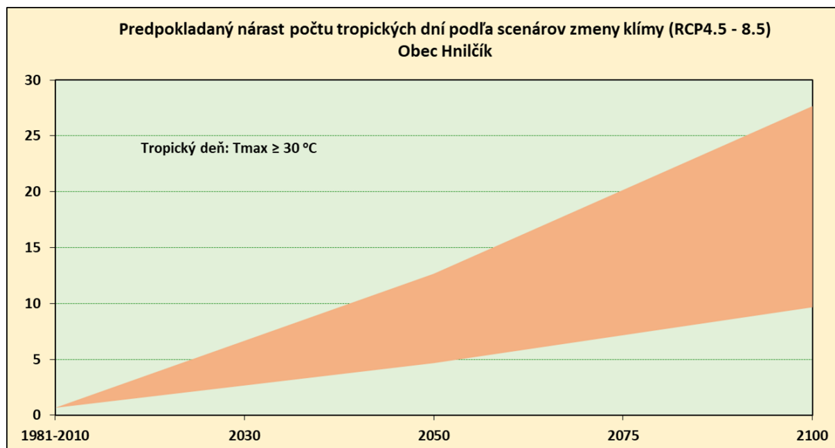
Obr.15 Predpokladaný nárast počtu tropických dní v obci Hnilčik podľa RCP scenárov
