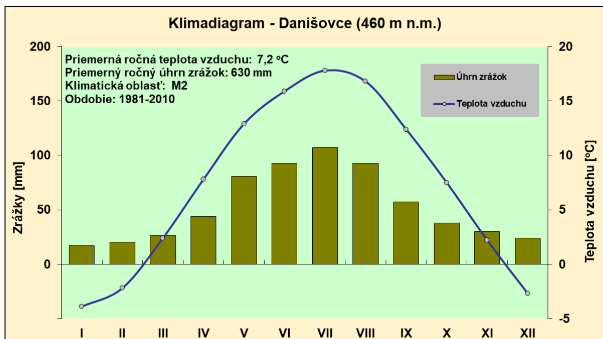
Obr.15 Klimadiagram obce Danišovce - súčasné klimatické podmienky (1981-2010)
