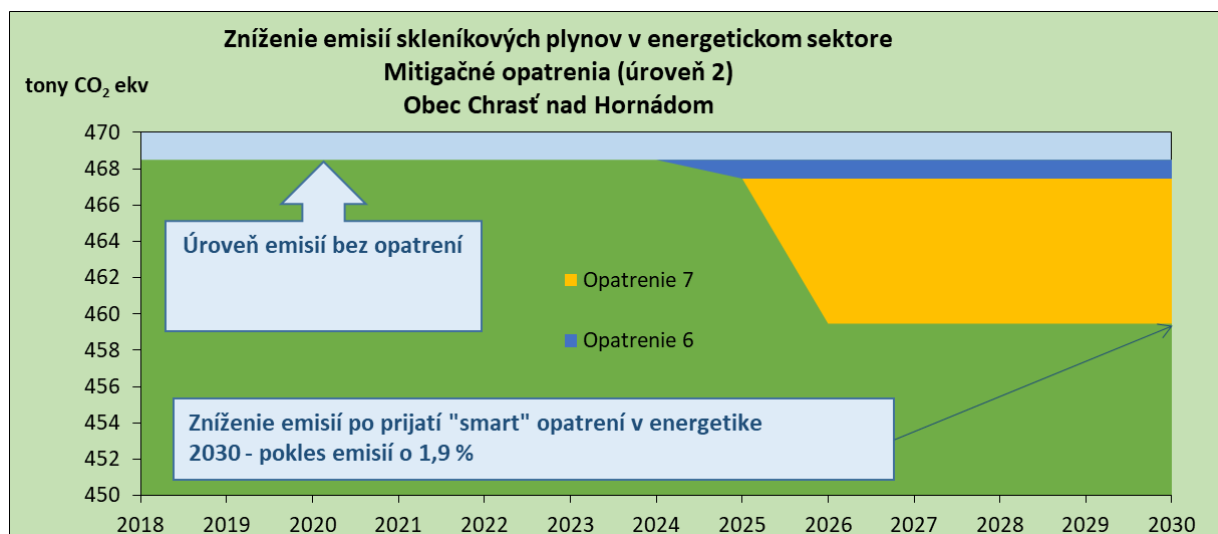
Obr.10 Zníženie emisií skleníkových plynov na báze prijatých mitigačných „smart“ opatrení – obec Chrást nad Hornádom
