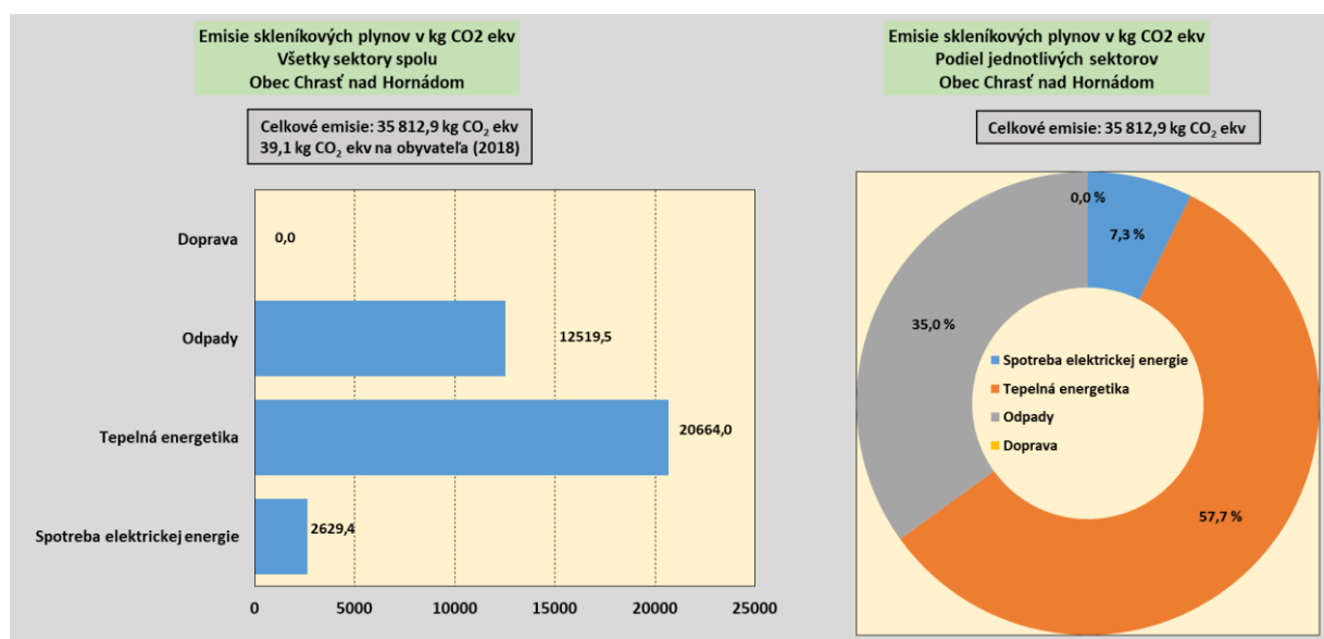
Obr.4 Podiel jednotlivých sektorov na celkových emisiách skleníkových plynov – verejný sektor obec Chrást nad Hornádom
