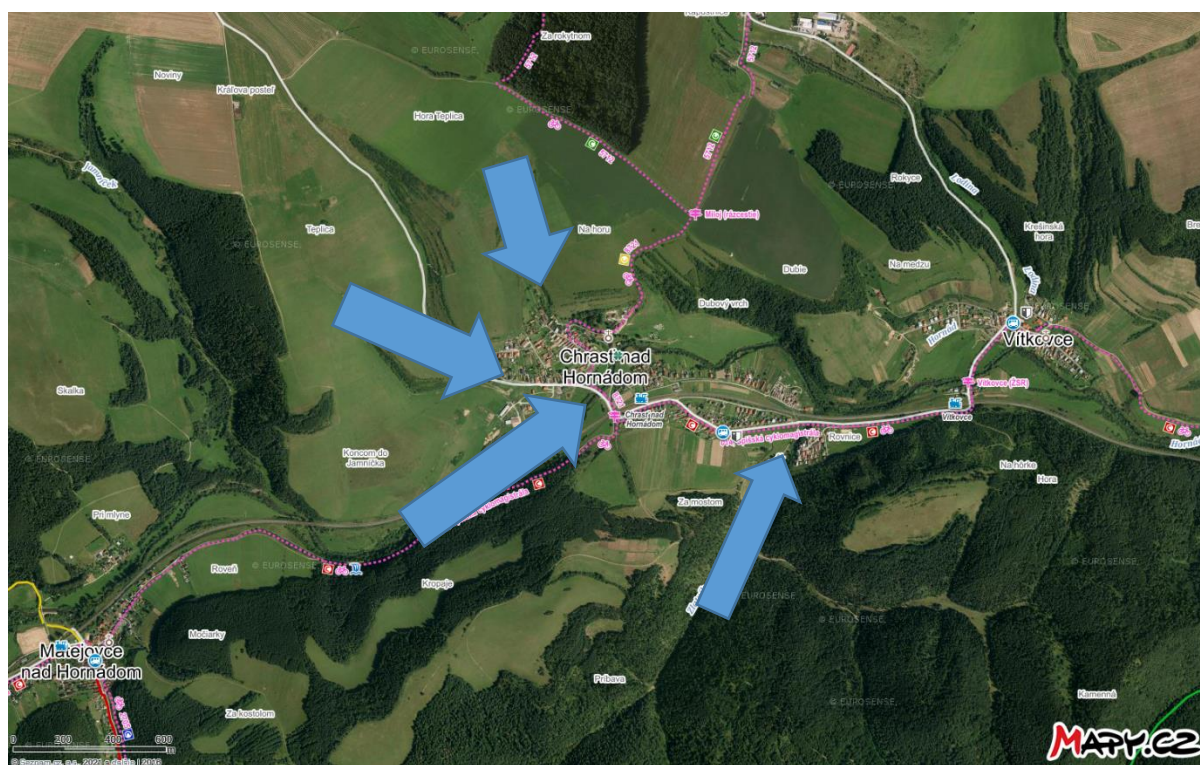
Obr.17 Nebezpečné smery bleskových záplav v lokalite obce Chrást nad Hornádom
