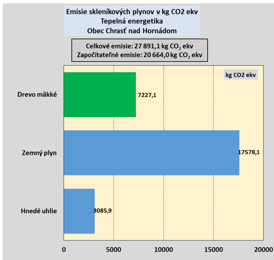
Obr.3 Emisie oxidu uhličitého (CO 2 ekv) v kg pre obecné budovy – obec Chrást nad Hornádom
