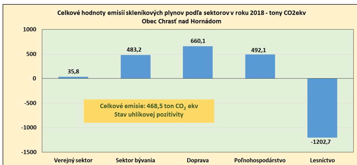
Obr.6 Celkové emisie skleníkových plynov v tonách CO 2 ekv za rok 2018 – obec Chrást nad Hornádom
