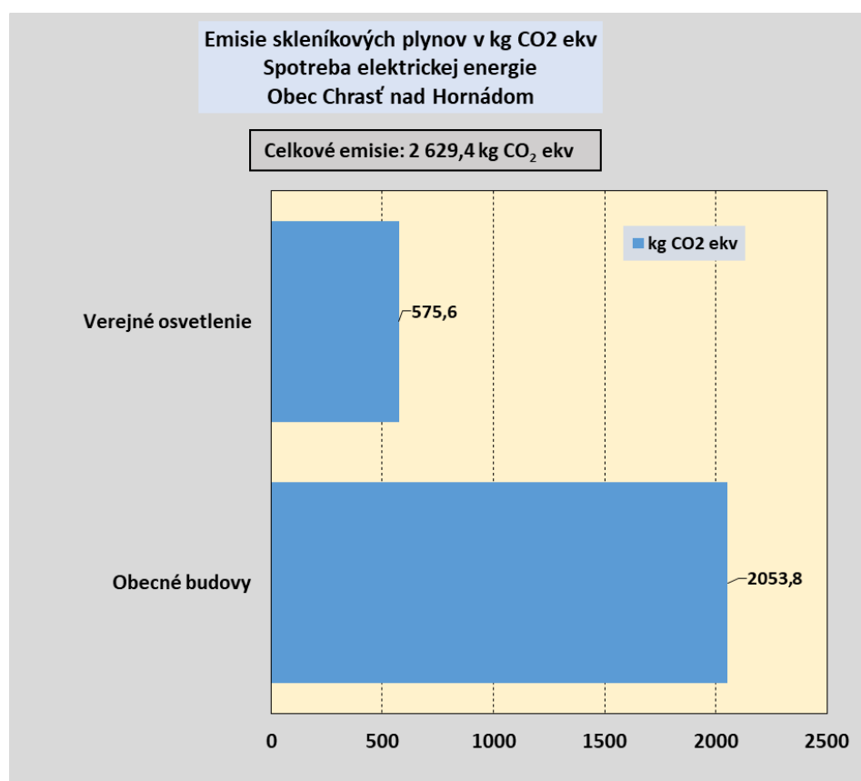
Obr.2 Emisie oxidu uhličitého (CO 2 eqv) v kg pre obecné budovy – obec Chrást nad Hornádom
