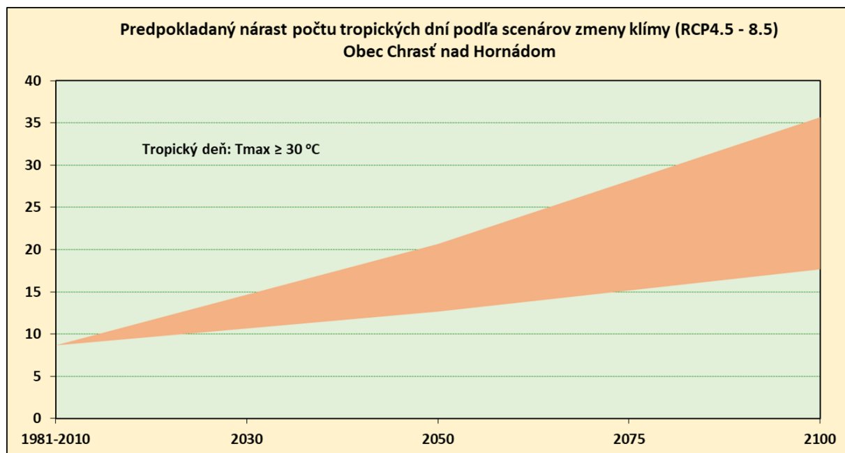
Obr.16 Predpokladaný nárast počtu tropických dní v obci Chrást nad Hornádom podľa RCP scenárov
