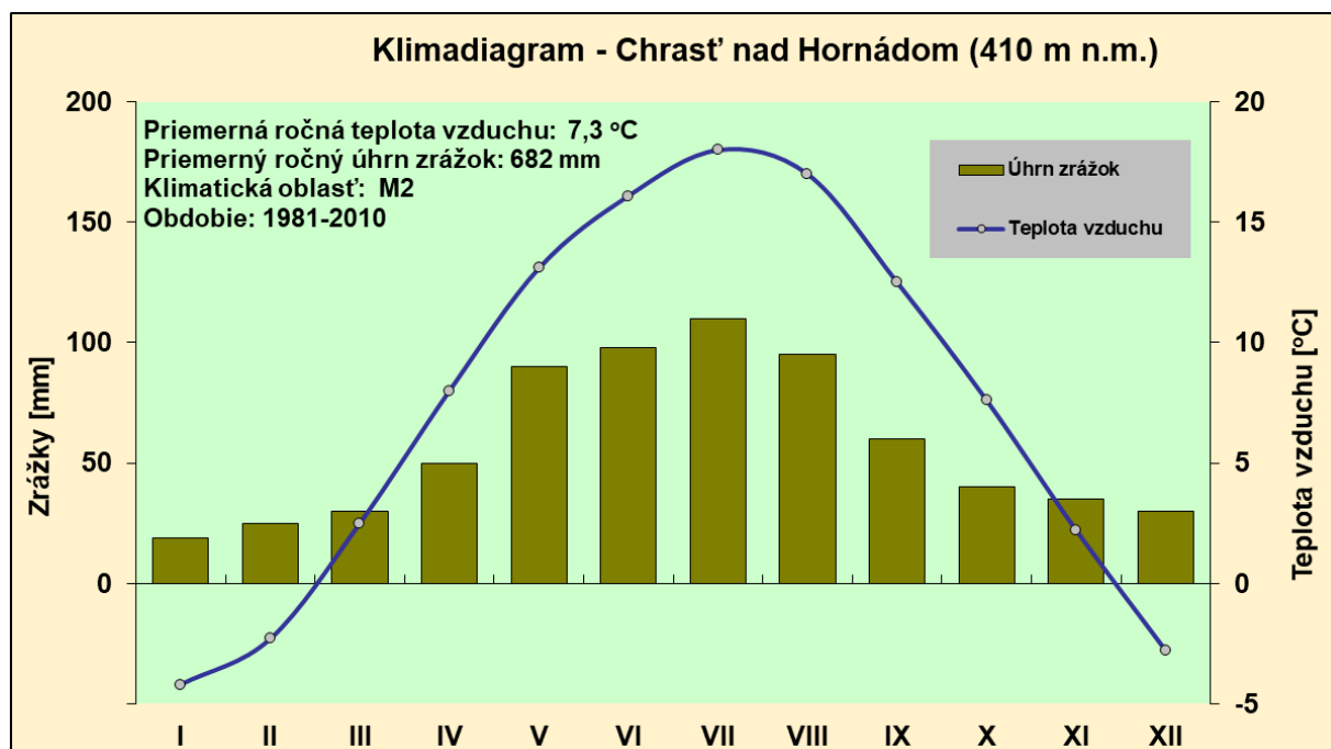
Obr.15 Klimadiagram obce Chrást nad Hornádom - súčasné klimatické podmienky (1981-2010)
