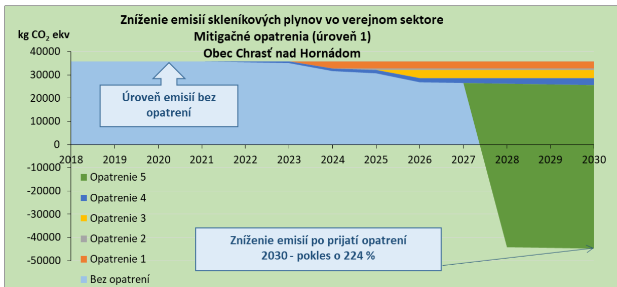
Obr.9 Zníženie emisií skleníkových plynov na báze prijatých mitigačných opatrení – obec Chrást nad Hornádom
