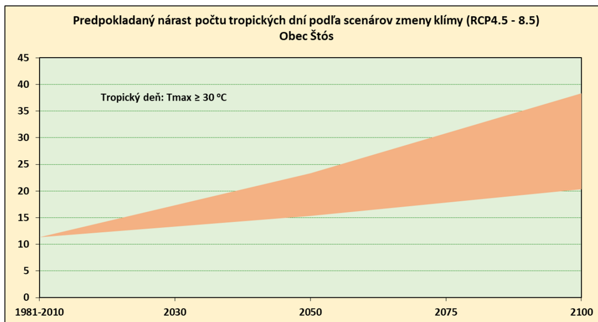
Obr.15 Predpokladaný nárast počtu tropických dní v obci Štós podľa RCP scenárov
