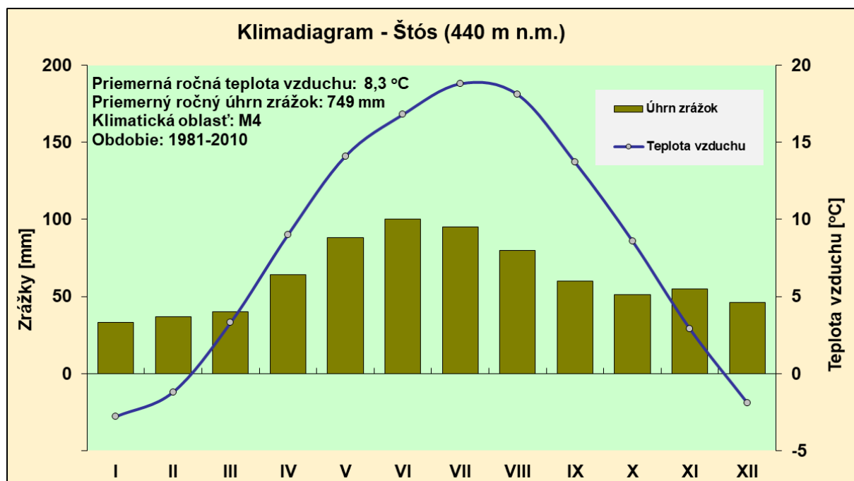
Obr.14 Klimadiagram obce Štós - súčasnú klimatické podmienky (1981-2010)
