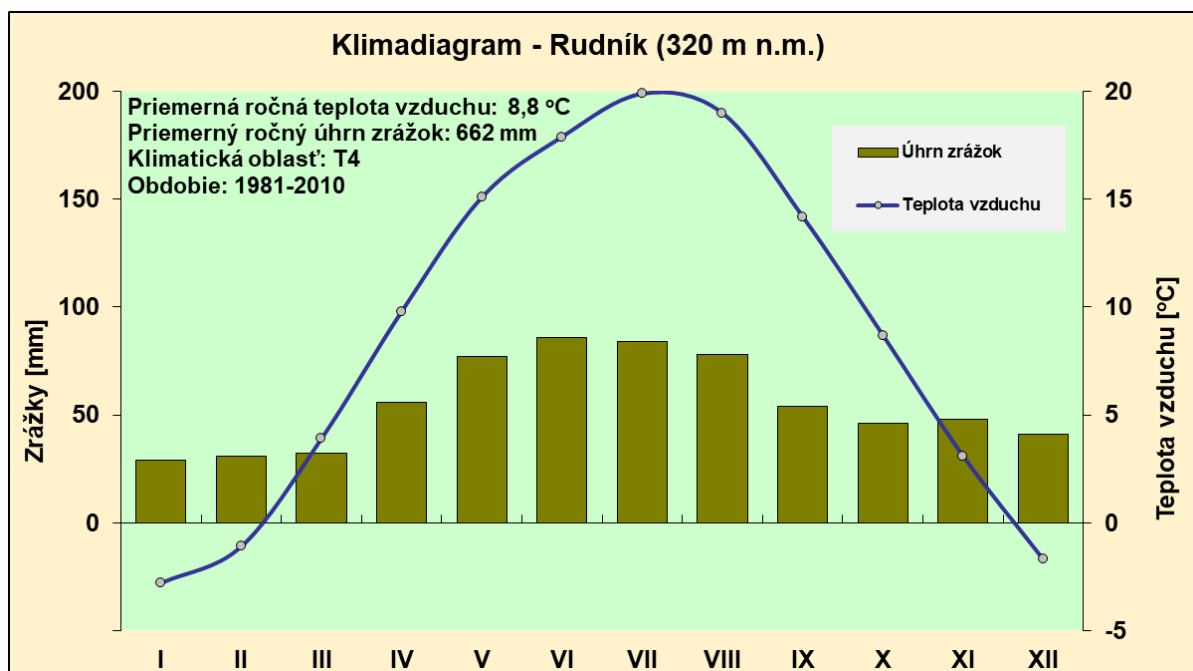
Obr.15 Klimadiagram obce Rudník - súčasné klimatické podmienky (1981-2010)
