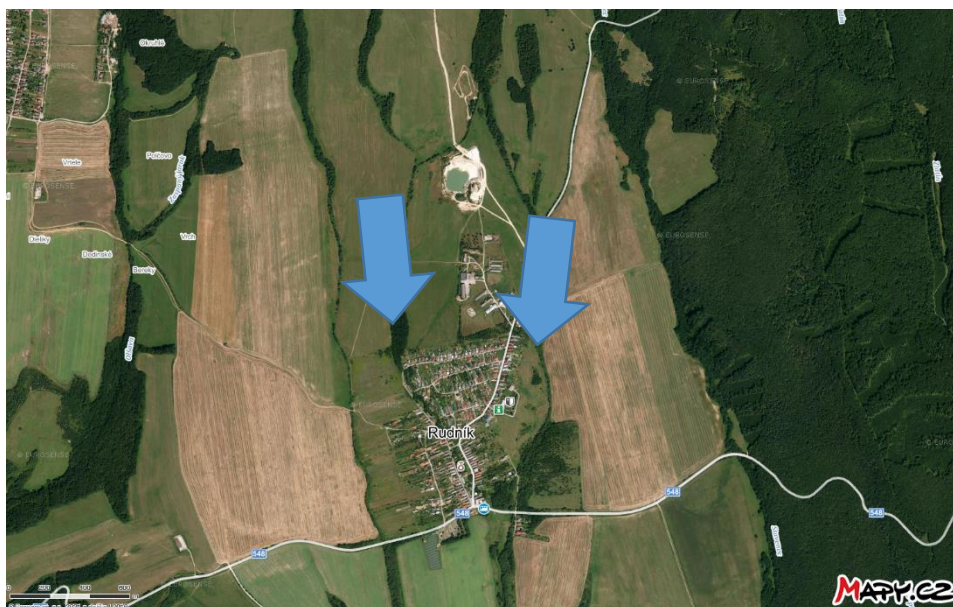
Obr.17 Nebezpečné smery bleskových záplav v lokalite obce Rudník
