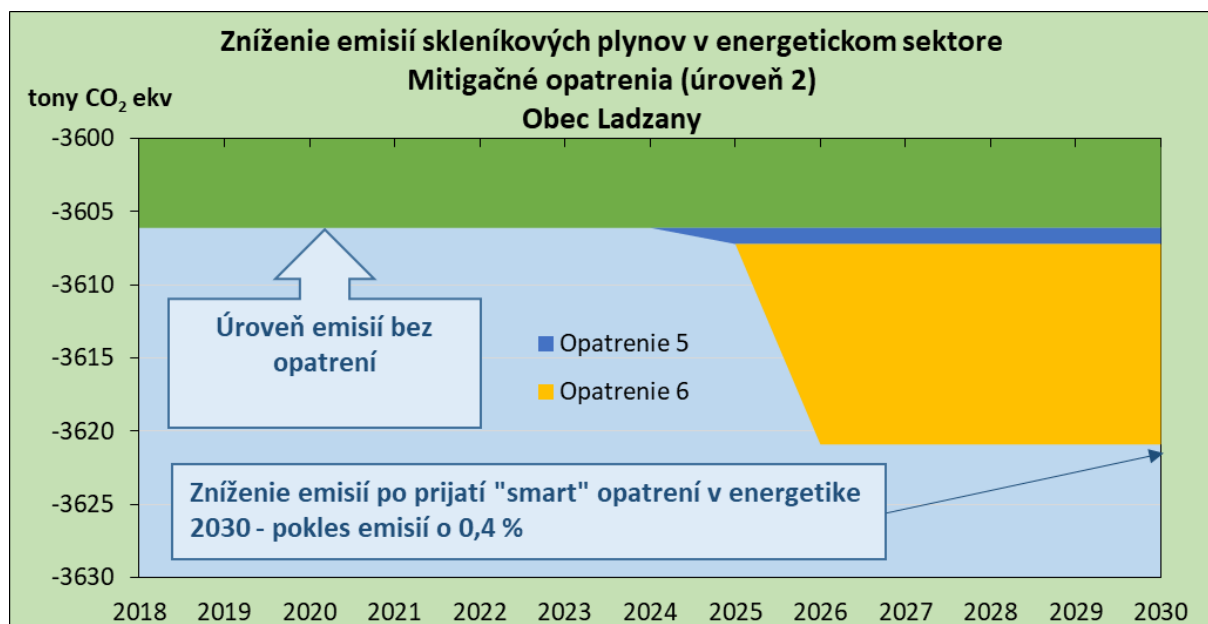
Obr.11 Zníženie emisií skleníkových plynov na báze prijatých mitigačných opatrení – obec Ladzany
