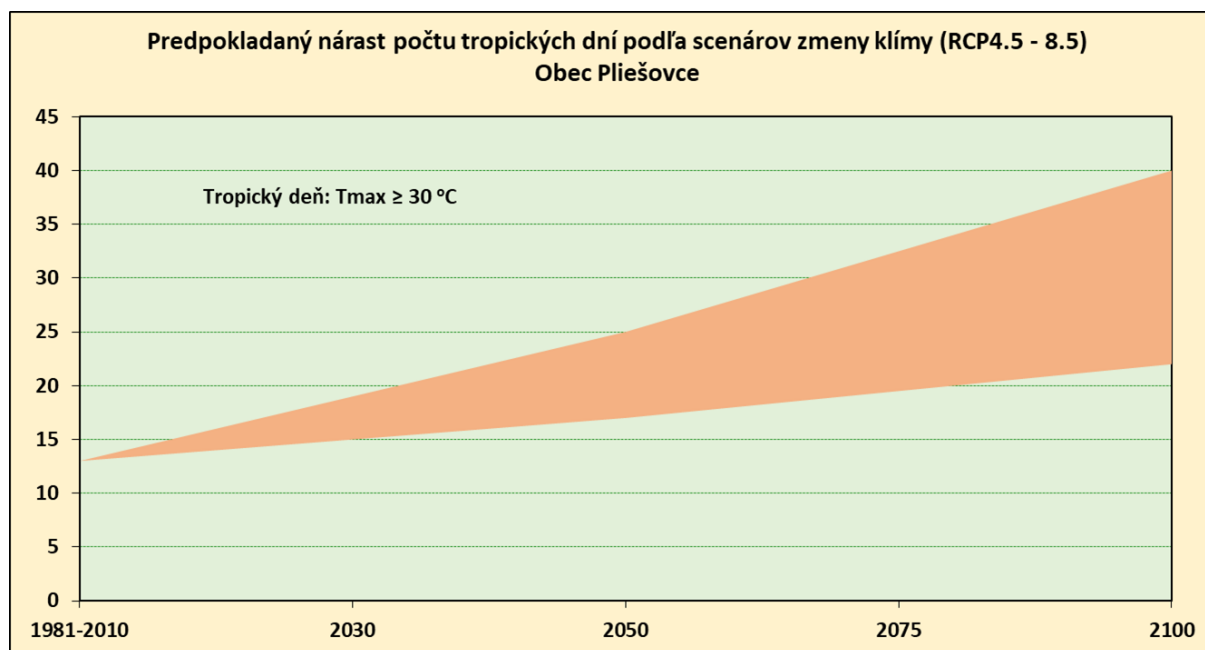
Obr.16 Predpokladaný nárast počtu tropických dní v obci Ladzany podľa RCP scenárov
