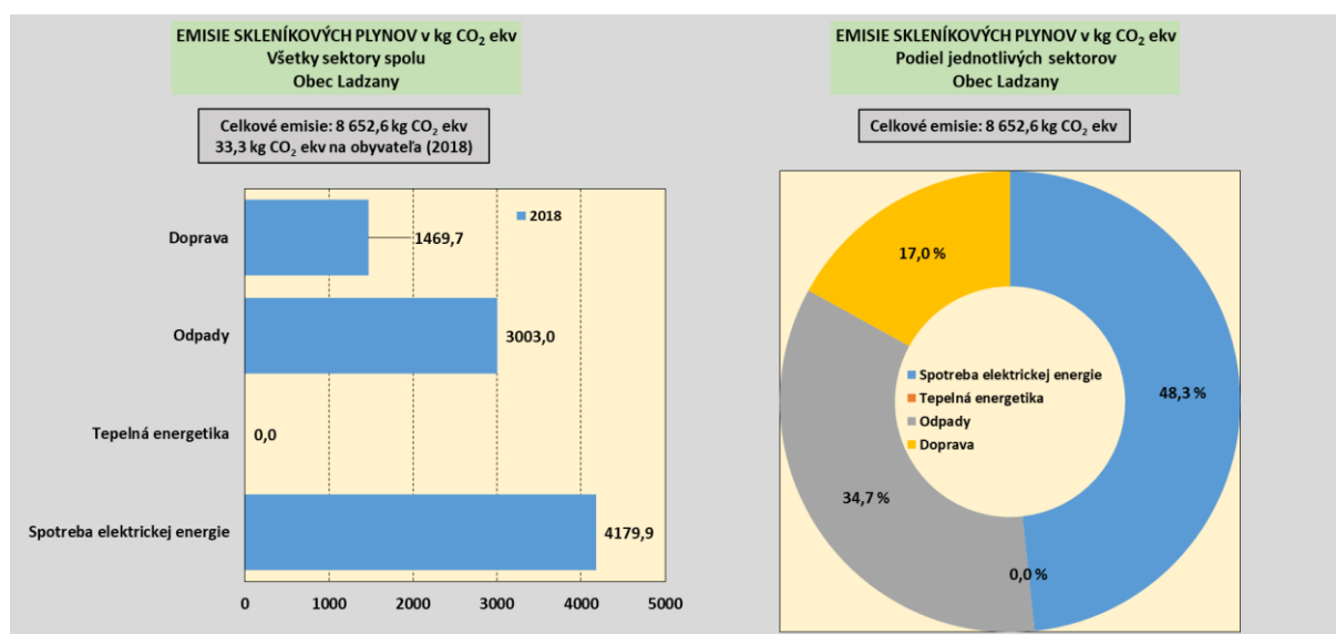
Obr.3 Podiel jednotlivých sektorov na celkových emisiách skleníkových plynov – verejný sektor obec Ladzany
