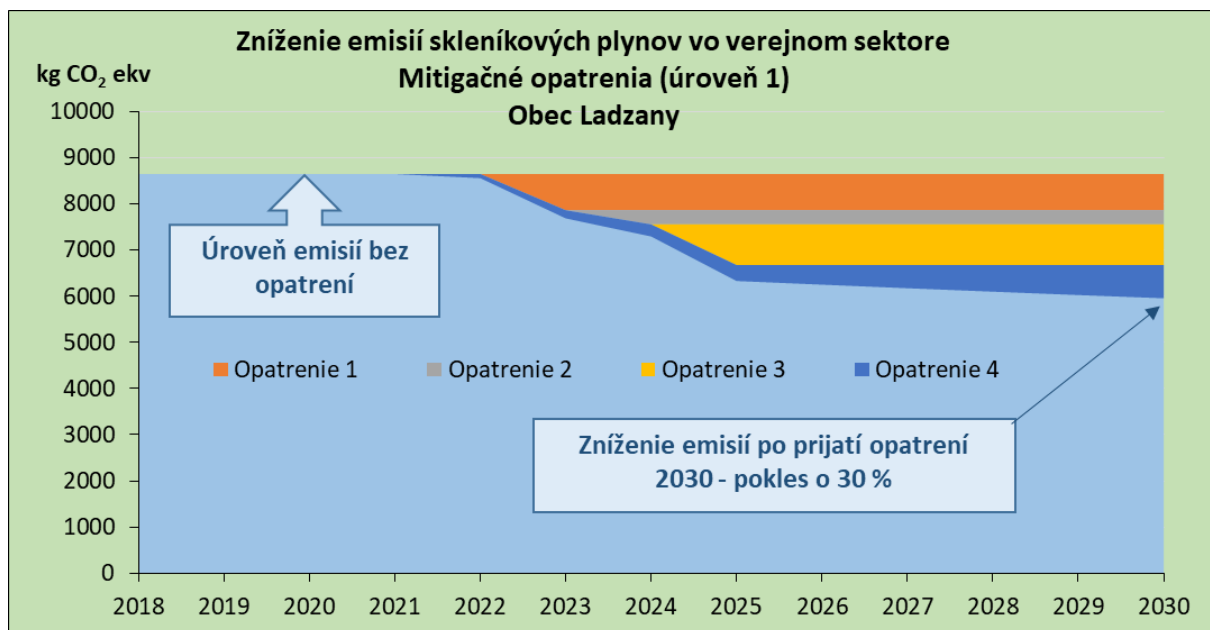
Obr.10 Zníženie emisií skleníkových plynov na báze prijatých mitigačných opatrení – obec Ladzany
