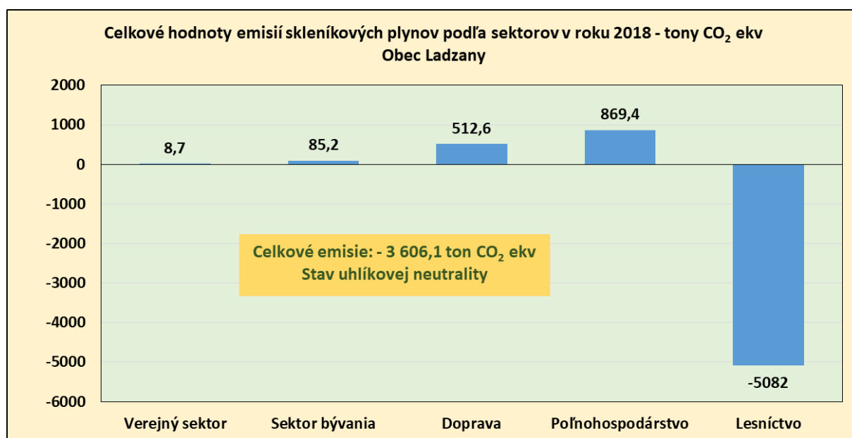
Obr.6 Celkové emisie skleníkových plynov v tonách CO 2 ekv za rok 2018 – obec Ladzany
