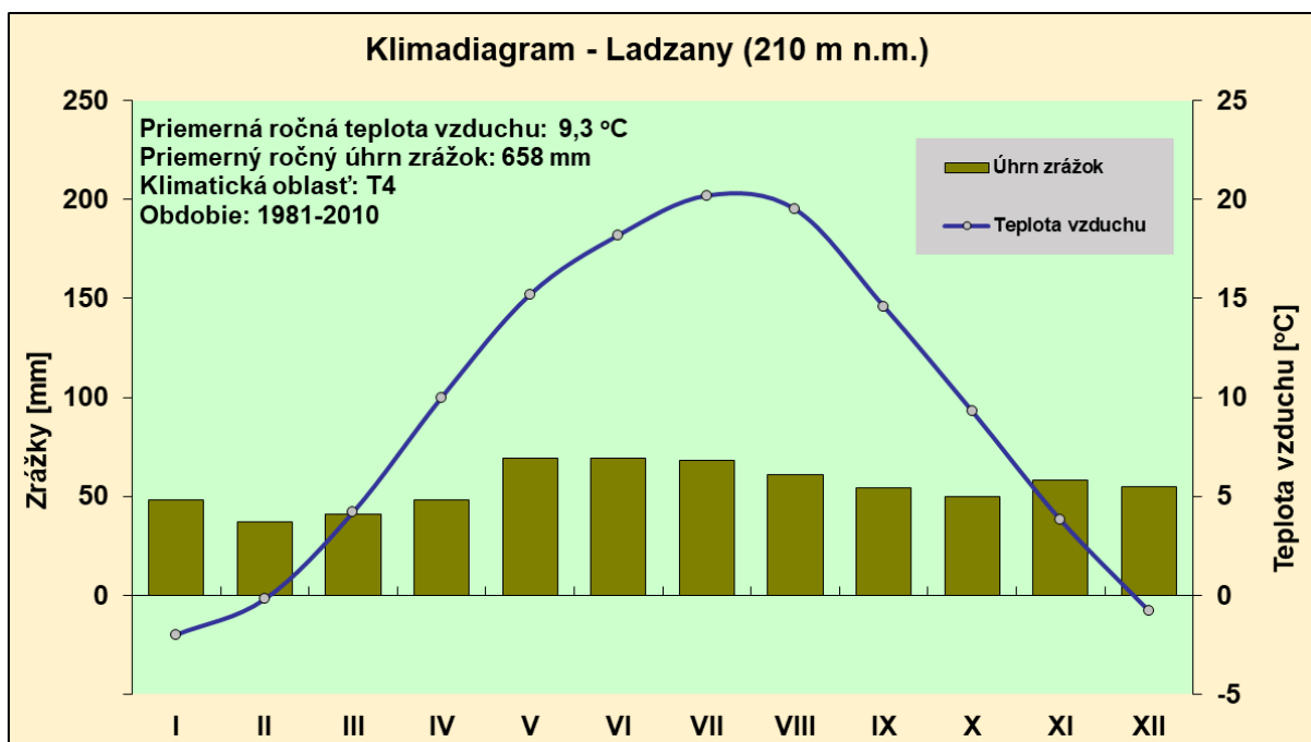
Obr.15 Klimadiagram obce Ladzany - súčasné klimatické podmienky (1981-2010)
