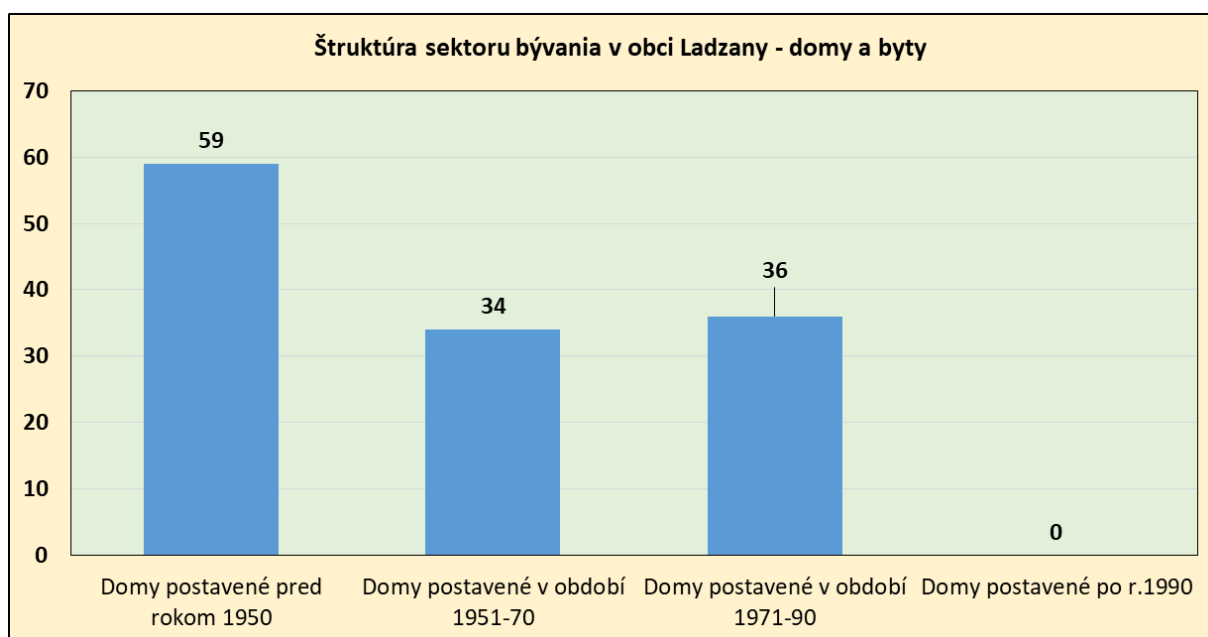
Obr.4 Štruktúra sektoru bývania v obci Ladzany – domy a byty
