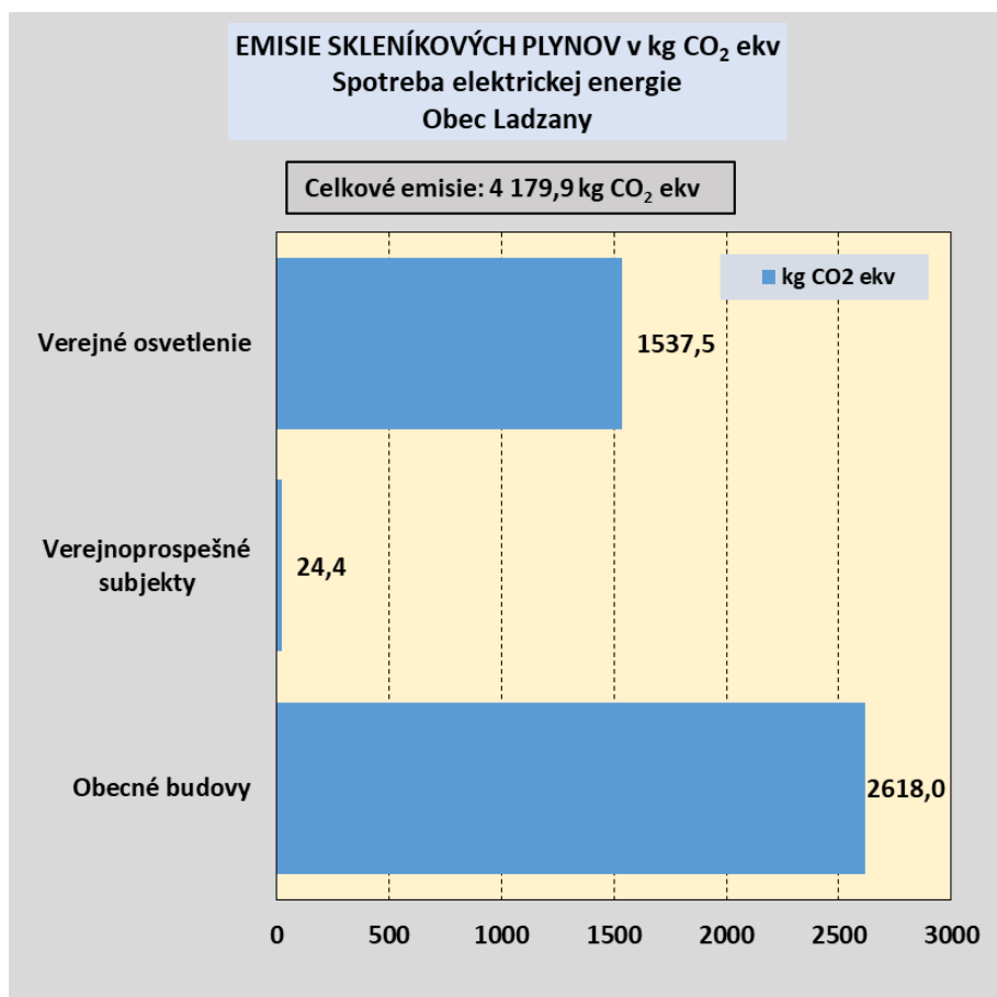
Obr.2 Emisie oxidu uhličitého (CO 2 ekv) v kg pre obecné budovy zo spotreby elektrickej energie – obec Ladzany
