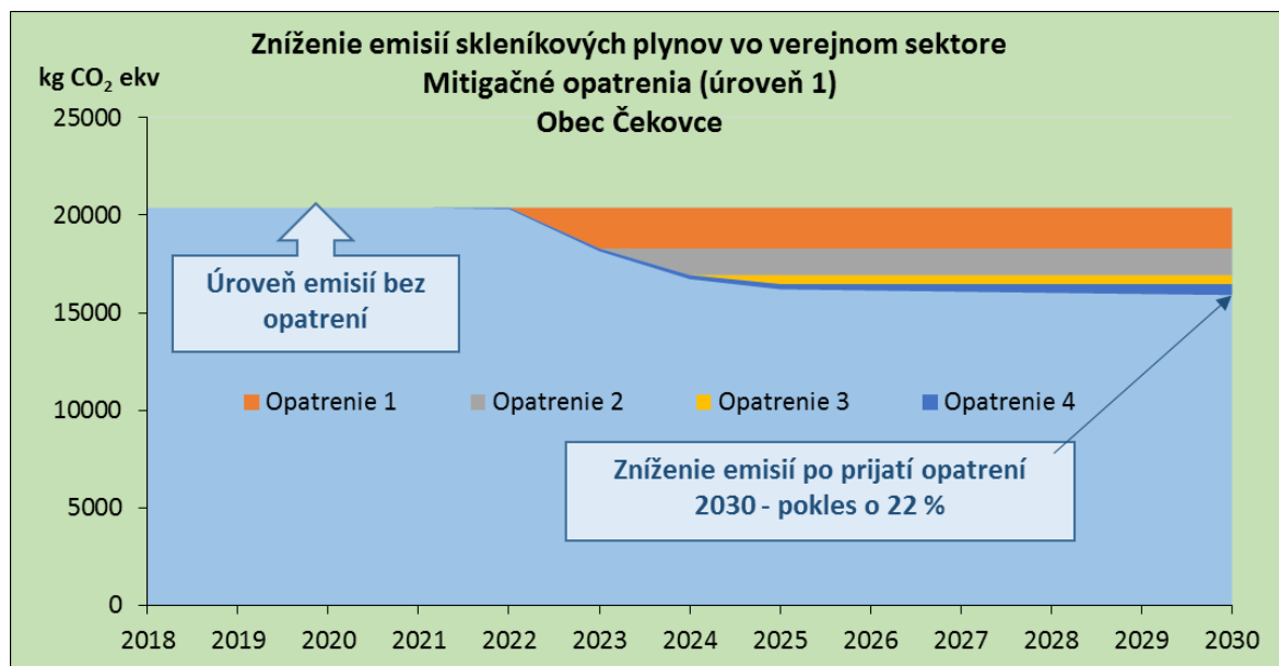
Obr.9 Zníženie emisií skleníkových plynov na báze prijatých mitigačných opatrení – obec Čekovce
