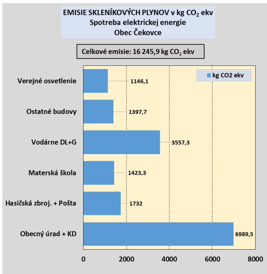
Obr.2 Emisie oxidu uhličitého (CO 2 ekv) v kg pre obecné budovy – obec Čekovce
