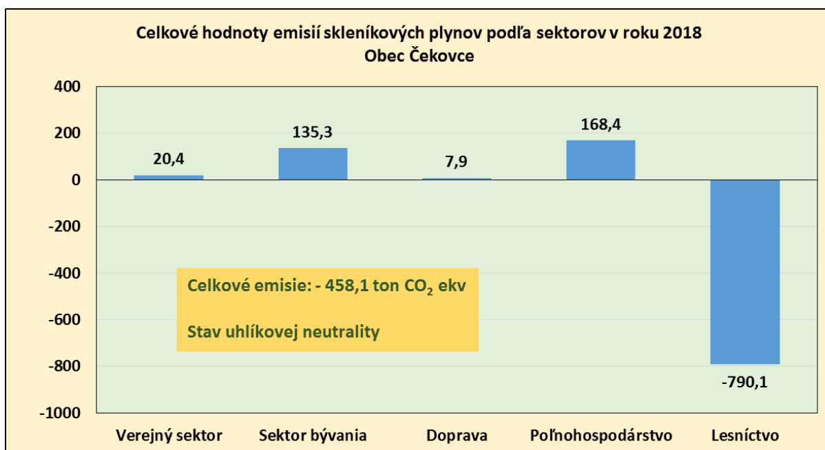
Obr.6 Celkové emisie skleníkových plynov v tonách CO 2 ekv za rok 2018 – obec Čekovce
