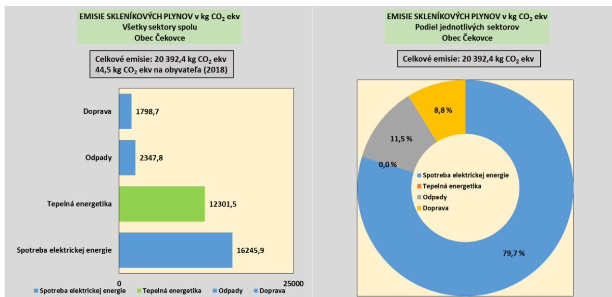
Obr.3 podiel jednotlivých sektorov na celkových emisiách skleníkových plynov – verejný sektor obec Čekovce
