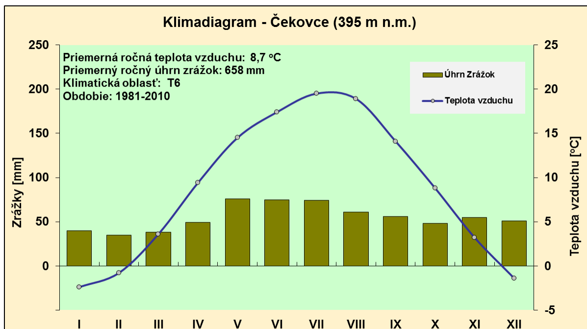
Obr.14 Klimadiagram obce Čekovce - súčasné klimatické podmienky (1981-2010)
