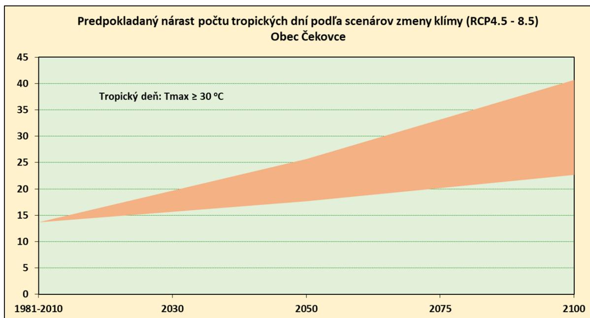
Obr.15 Predpokladaný nárast počtu tropických dní v obci Čekovce podľa RCP scenárov
