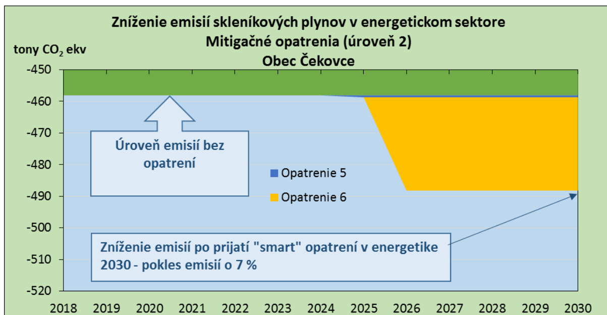
Obr.10 Zníženie emisií skleníkových plynov na báze prijatých mitigačných opatrení – obec Čekovce
