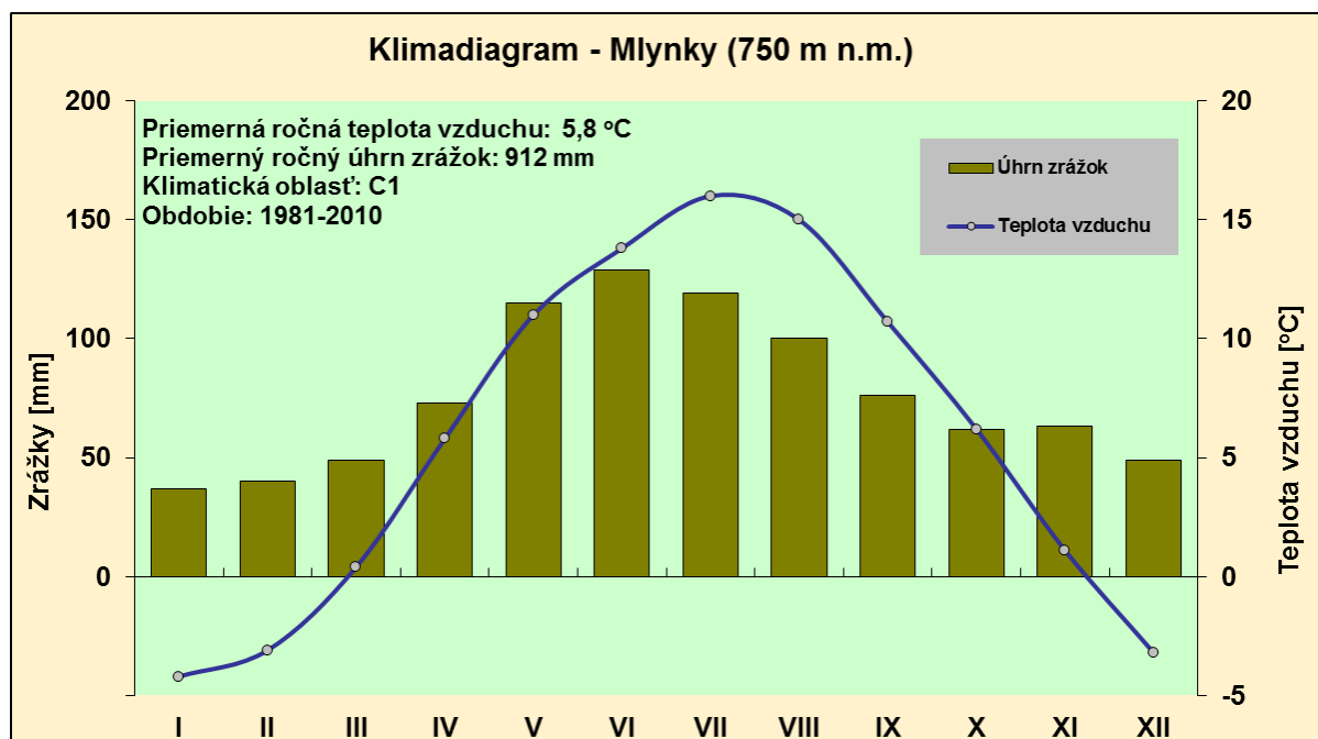
Obr.14 Klimadiagram obce Mlynky - súčasné klimatické podmienky (1981-2010)
