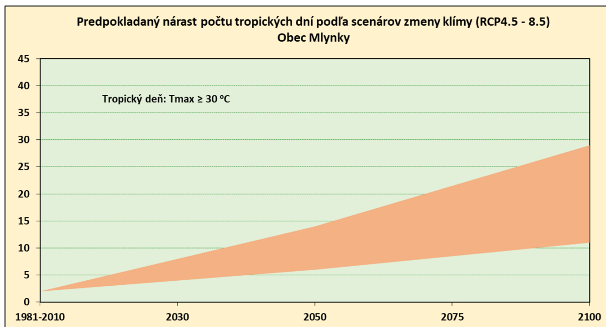
Obr.15 Predpokladaný nárast počtu tropických dní v obci Mlynky podľa RCP scenárov
