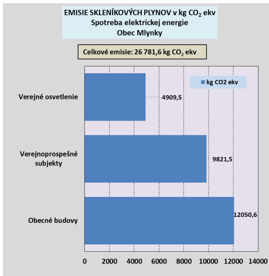
Obr.2 Emisie oxidu uhličitého (CO 2 ekv) v kg pre obecné budovy – obec Mlynky
