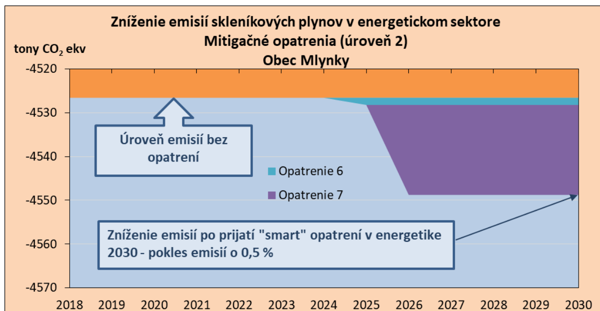
Obr.10 Zníženie emisií skleníkových plynov na báze prijatých mitigačných opatrení – obec Mlynky
