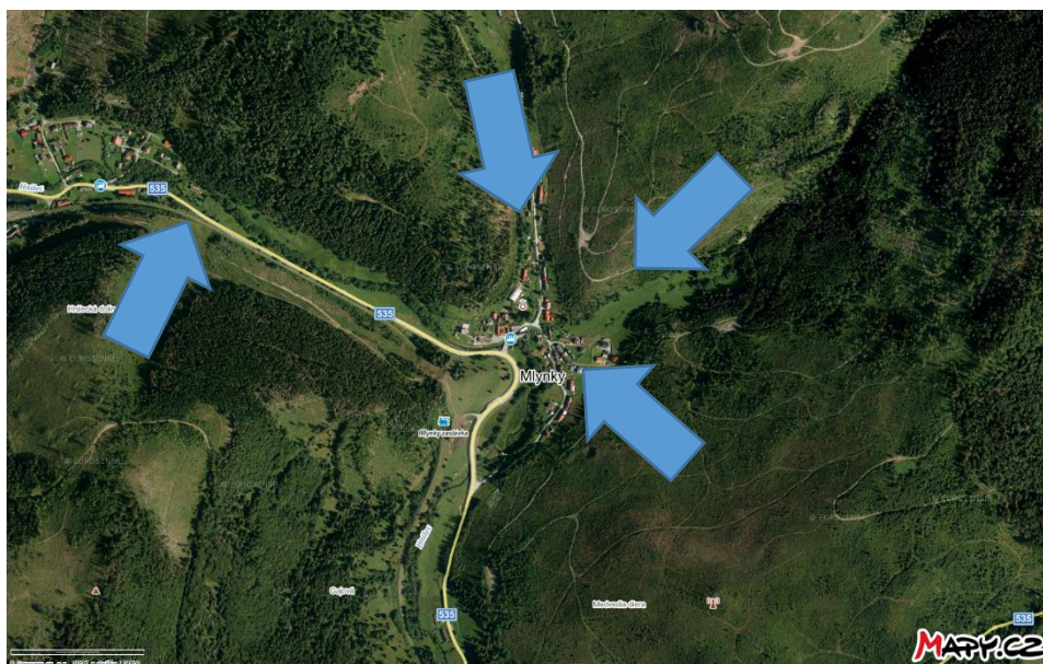
Obr.16 Nebezpečné smery bleskových záplav v lokalite obce Mlynky
