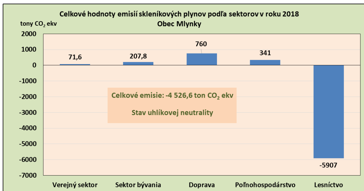
Obr.6 Celkové emisie skleníkových plynov v tonách CO 2 ekv za rok 2018 – obec Mlynky
