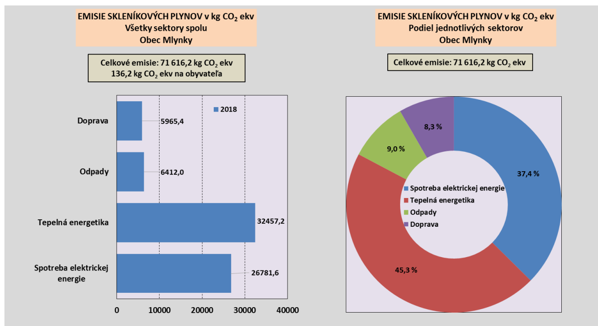
Obr.3 Podiel jednotlivých sektorov na celkových emisiách skleníkových plynov – verejný sektor obec Mlynky
