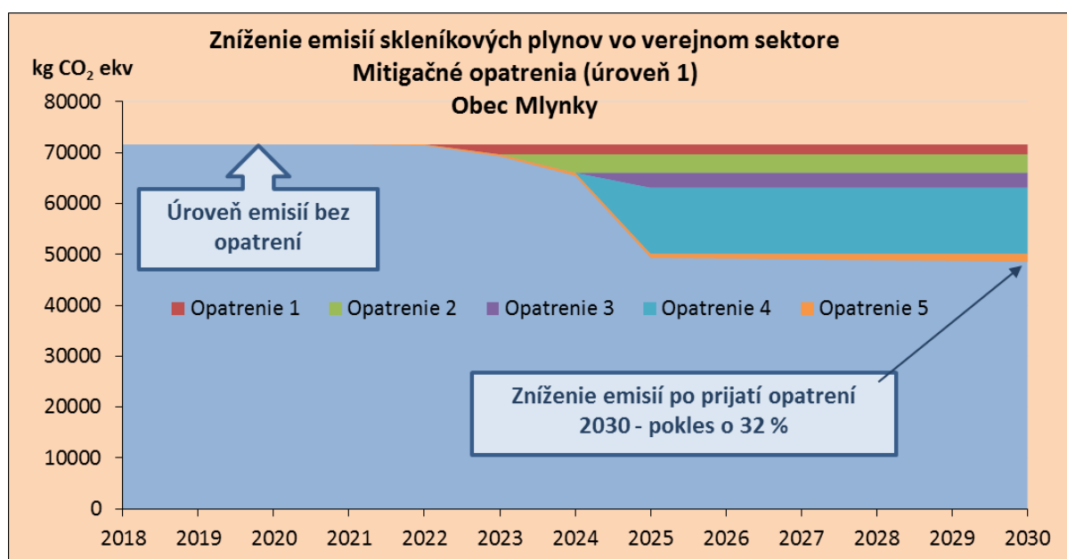
Obr.9 Zníženie emisií skleníkových plynov na báze prijatých mitigačných opatrení – obec Mlynky
