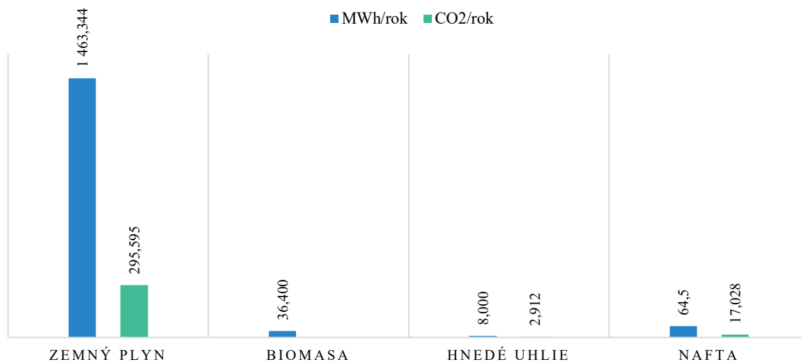
Graf 23 Množstvo spotrebovanej energie a produkcia emisii podľa typu paliva MZZO
