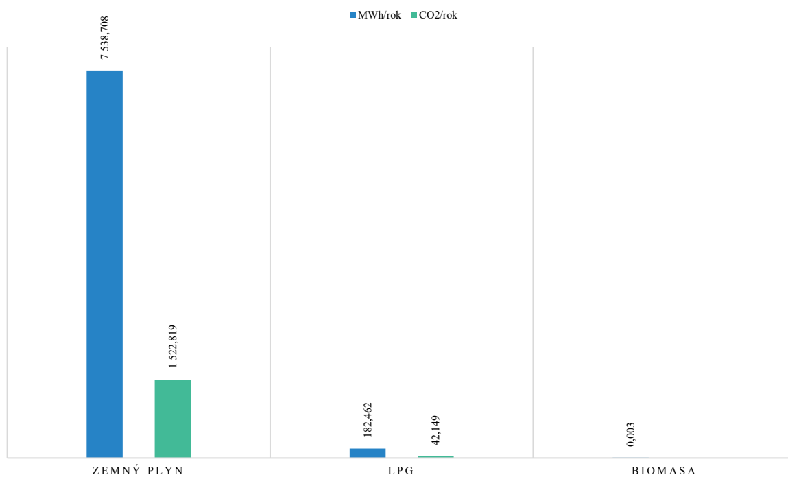
Graf 22 Množstvo spotrebovanej energie a produkcia emisii podľa typu paliva SZZO a VZZO
