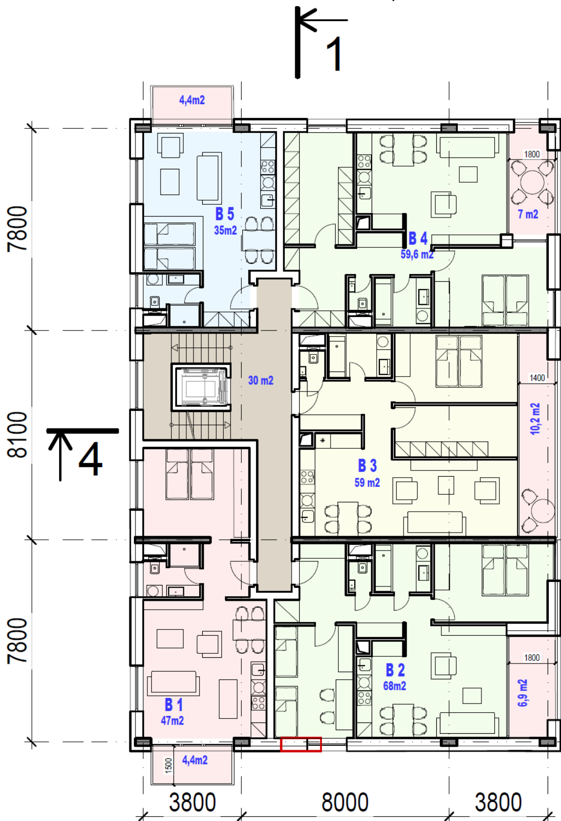
Obr. 6: Typové podlažie
