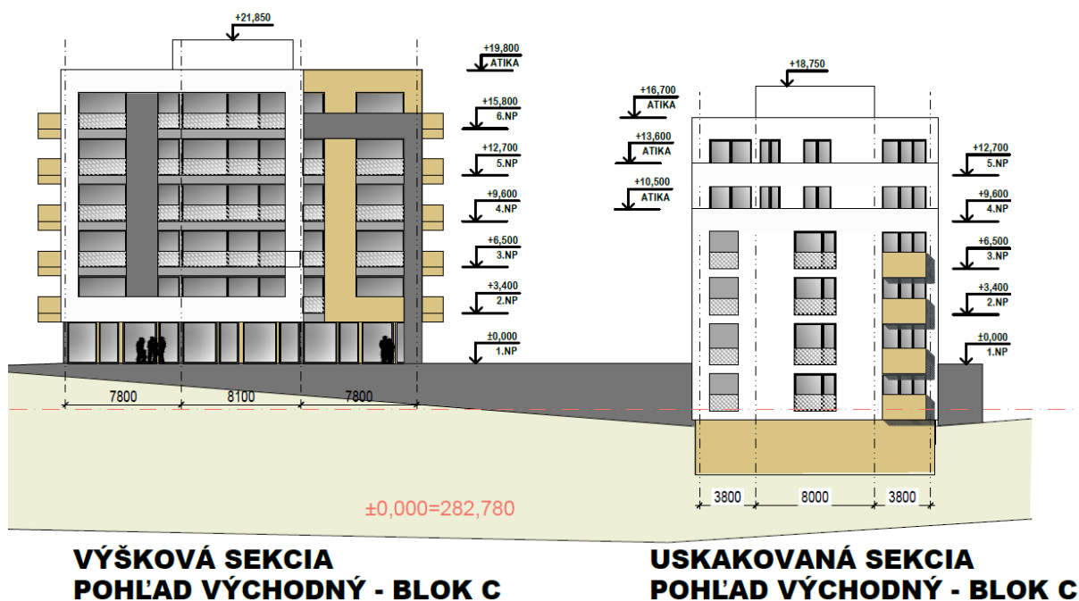
Obr. 7: Pohľady
