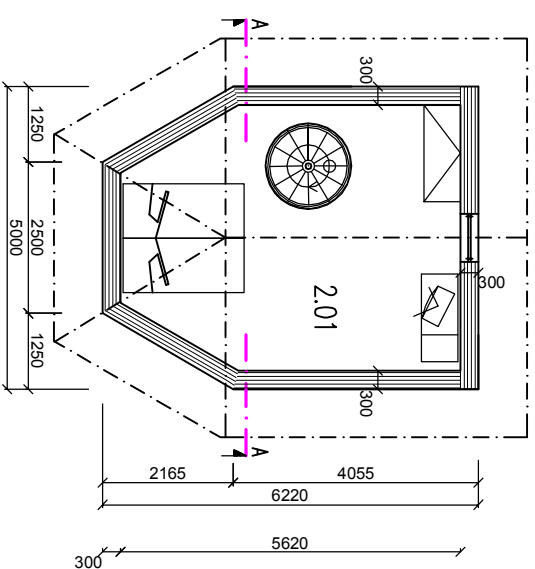
PÔDORYS PODKROVIA
