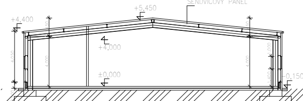
REZ B-B
