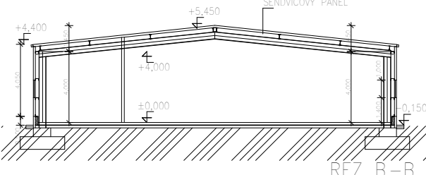
REZ B-B
