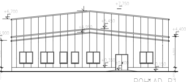
POHLAD P1
