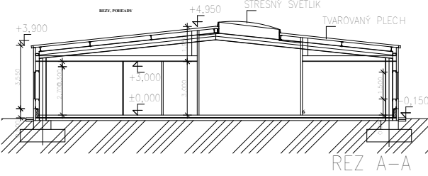
REZ A-A
