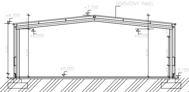
REZ C-C
