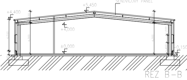
REZ A-A
