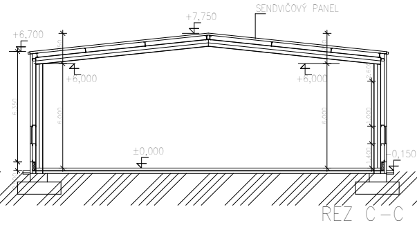
REZ C-C
