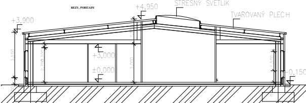
REZ A-A
