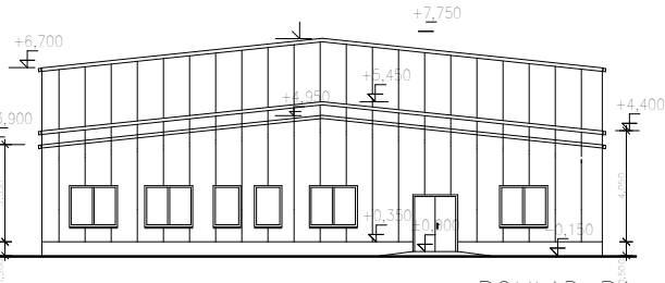
POHLAD P1
