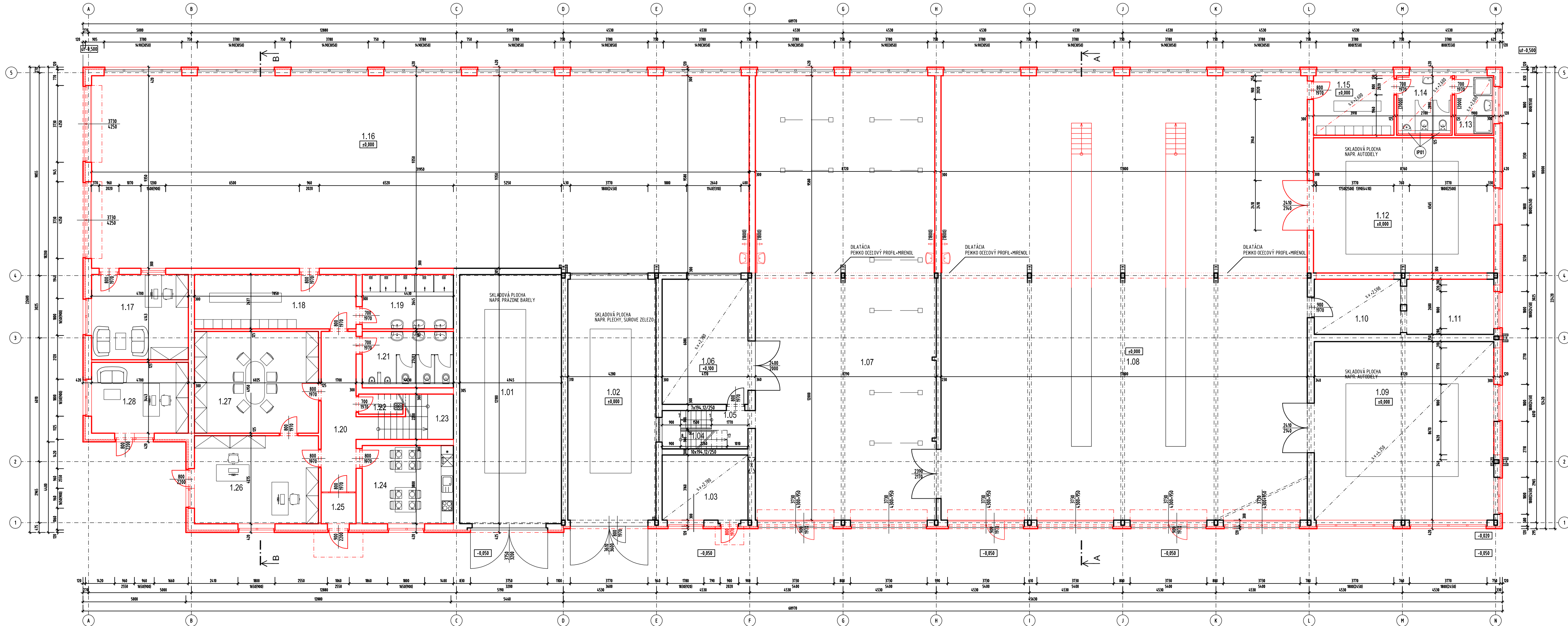
PÓDORYS PRÍZEMIA - NAVRHOVANÝ STAV M 1:75
