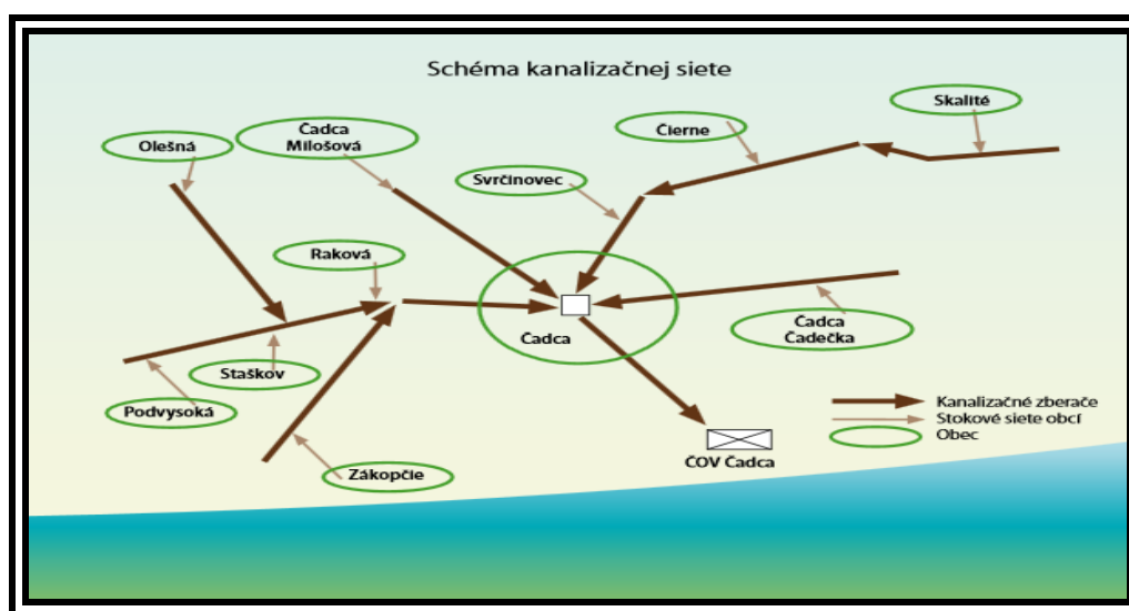
Obrázok 10 Schéma skupinovej kanalizačnej siete Čadca - ČOV Čadca
