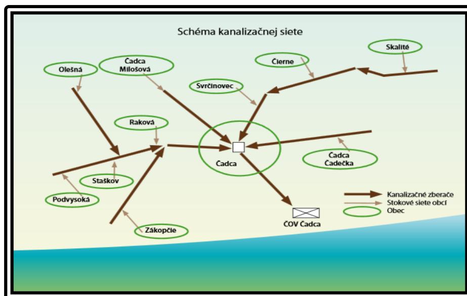
Obrázok 10 Schéma skupinovej kanalizačnej siete Čadca - ČOV Čadca
