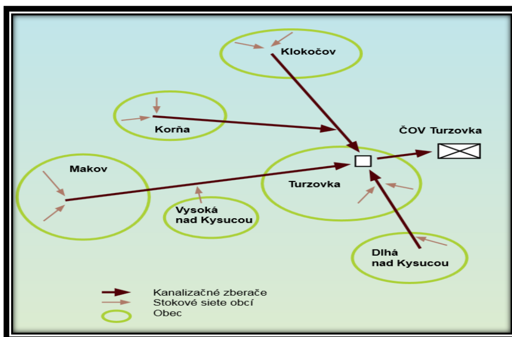
Obrázok 10 Schéma skupinovej kanalizačnej siete Turzovka - ČOV Turzovka
