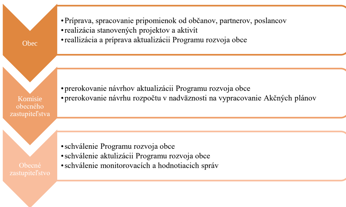
Obrázok 1 Matica zodpovednosti
