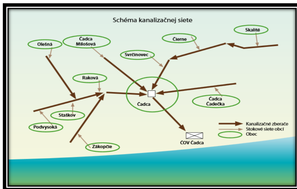
Obrázok 10 Schéma skupinovej kanalizačnej siete Čadca - ČOV Čadca
