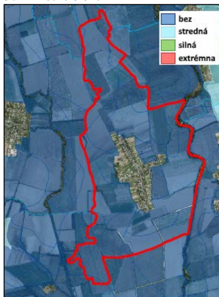
Obr. 2: Vodná erózia
