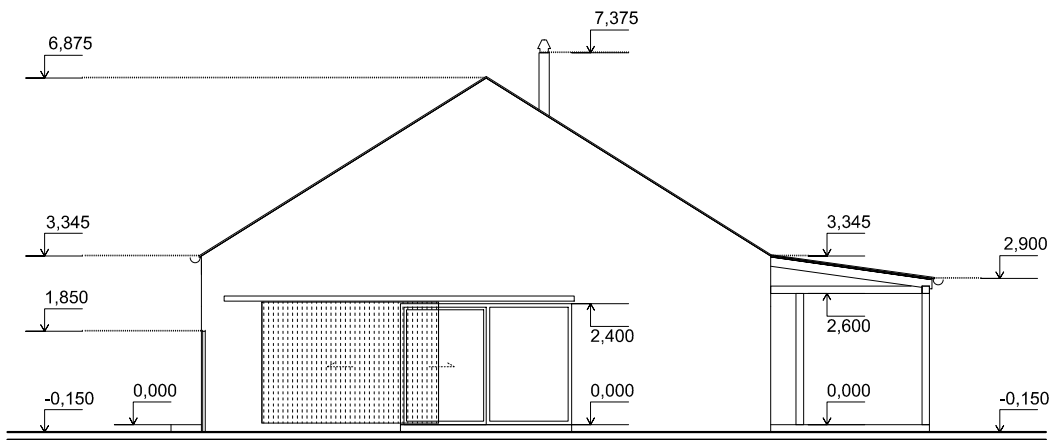
POHLAD SEVEROZÁPADNÝ SO 101
