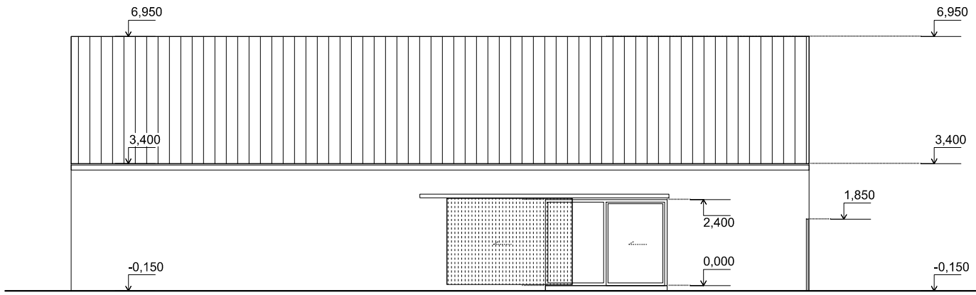
POHLAD JUHOVÝCHODNÝ SO 100
