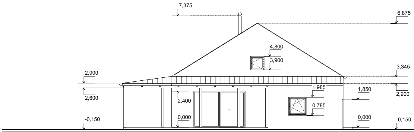
POHLAD JUHOVÝCHODNÝ SO 101
