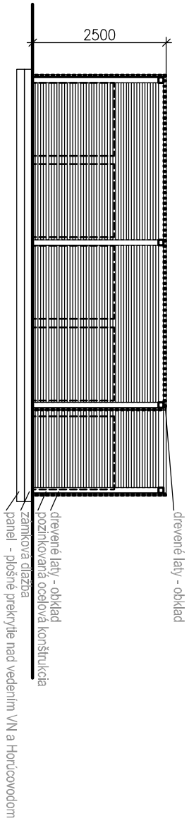
schematický rez
