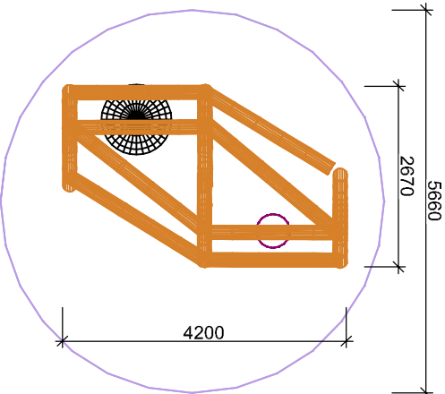
podorysná schéma
