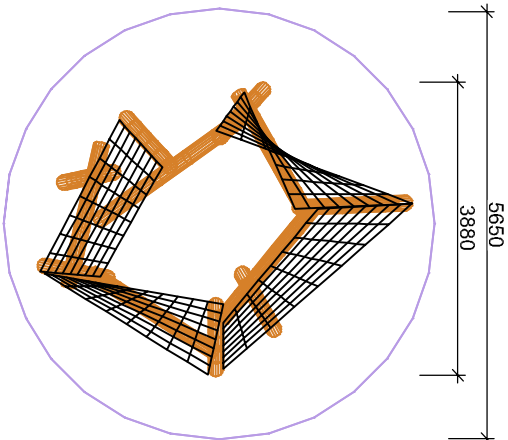
podorysná schéma
