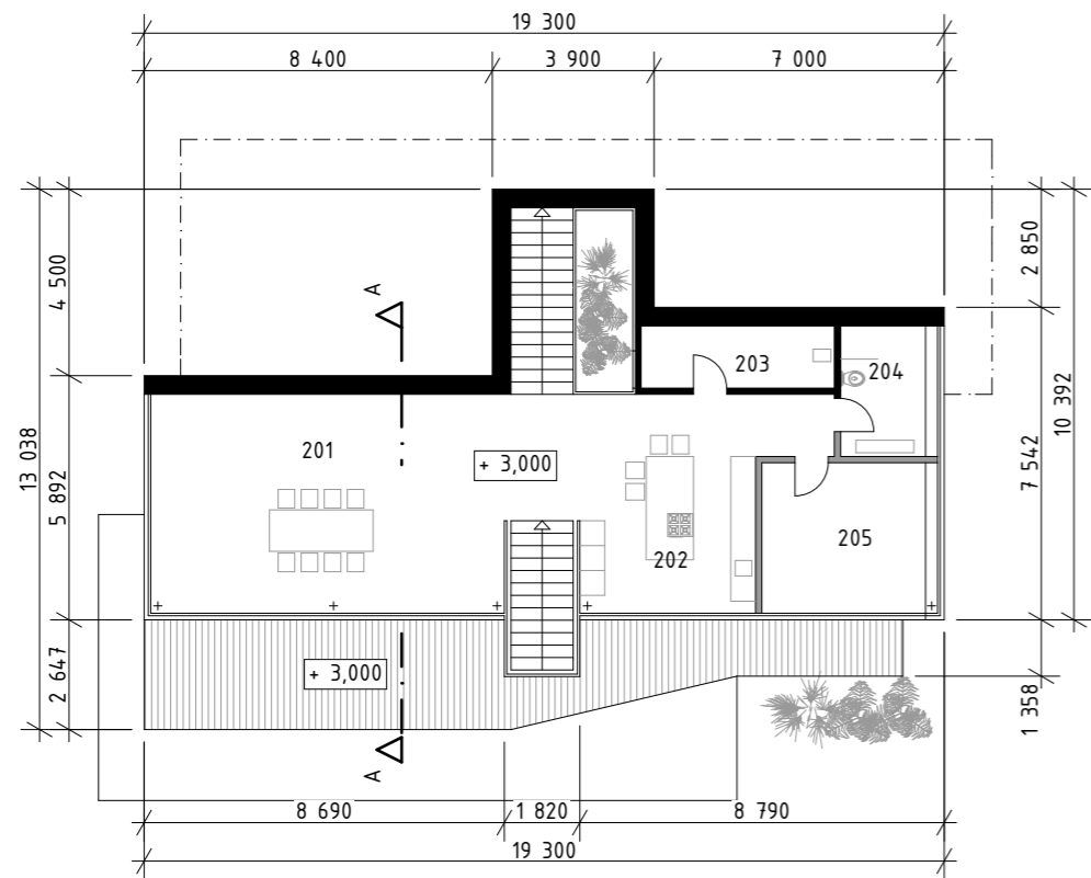
PÔDORYS 2.NP
