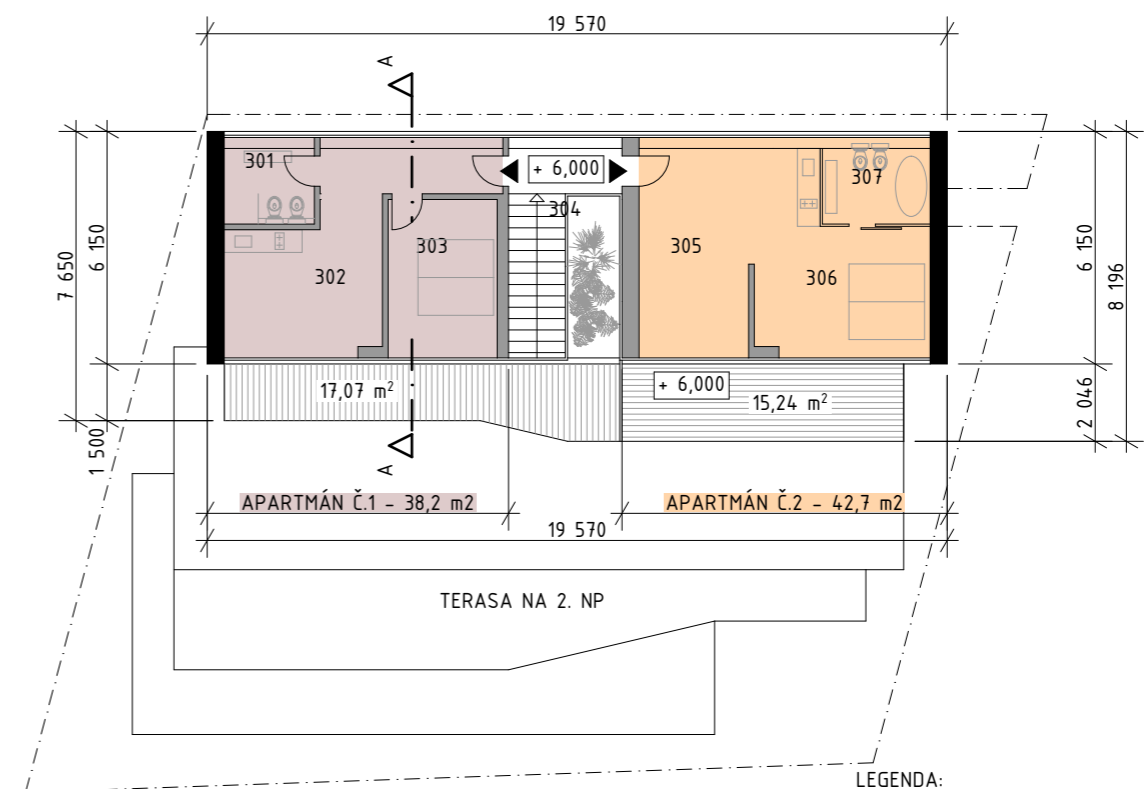
PÔDORYS 3.NP
