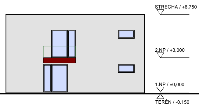
POHĽAD JUHOVÝCHODNÝ
