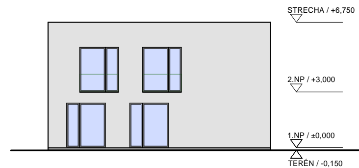
POHĽAD SEVEROZÁPADNÝ - ALT.2
