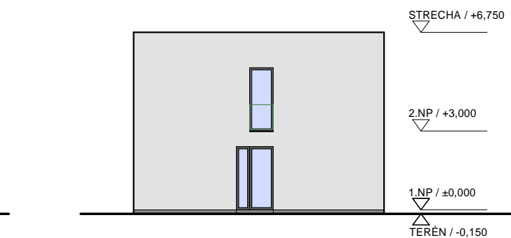
POHĽAD SEVEROVÝCHODNÝ - ALT.2
