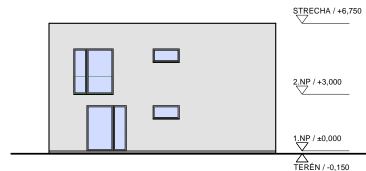
POHĽAD SEVEROZÁPADNÝ
