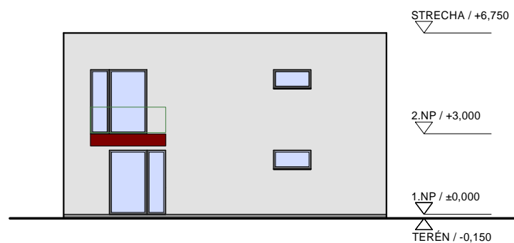
POHĽAD JUHOVÝCHODNÝ - ALT.2
