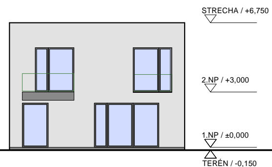
POHĽAD JUHOZÁPADNÝ
