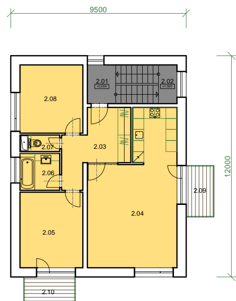
PÔDORYS 1.NP
