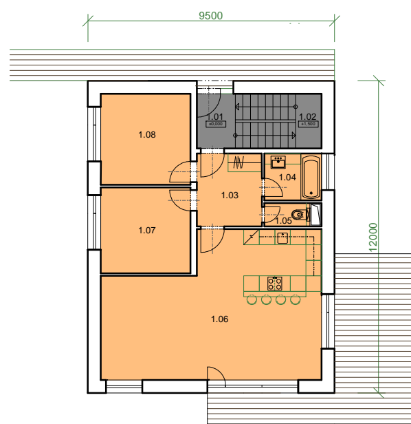
PÔDORYS 1.NP - ALT.2
