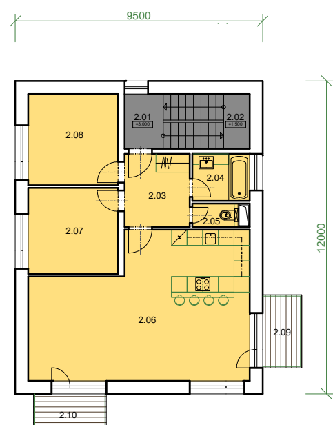
PÔDORYS 2.NP - ALT.2
