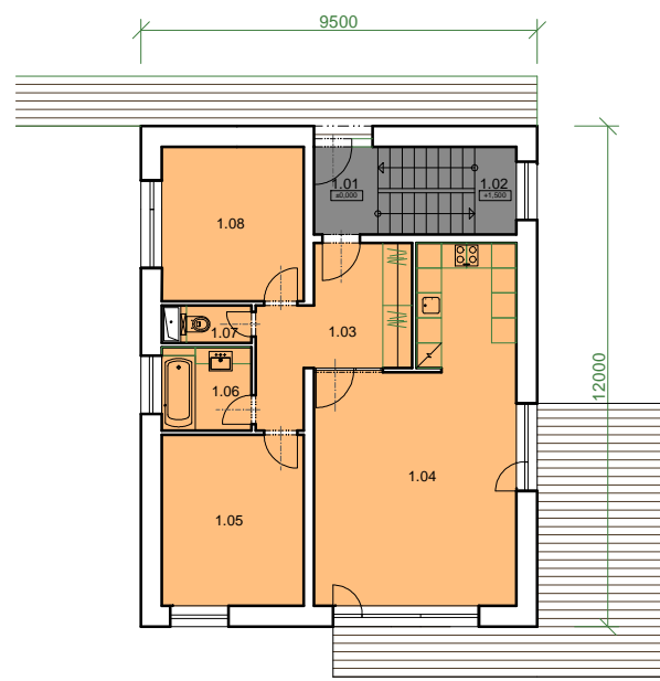
PÔDORYS 1.NP
