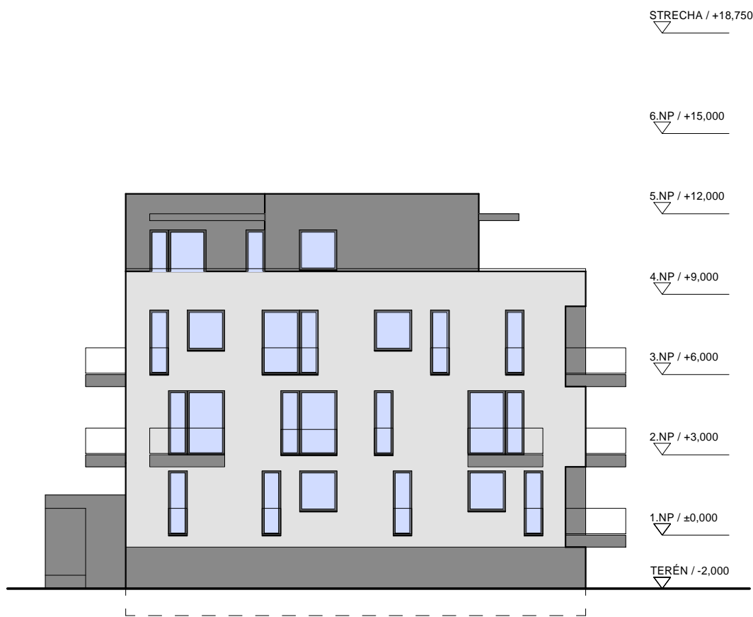
POHLAD SEVEROZÁPADNÝ
