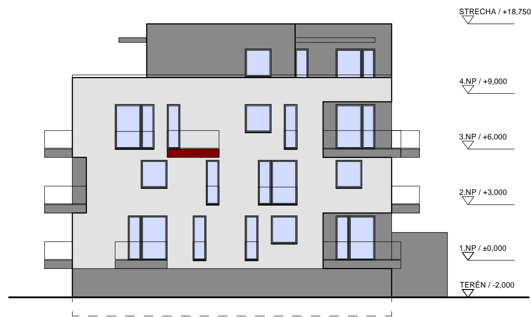
POHLAD JUHOVÝCHODNÝ
