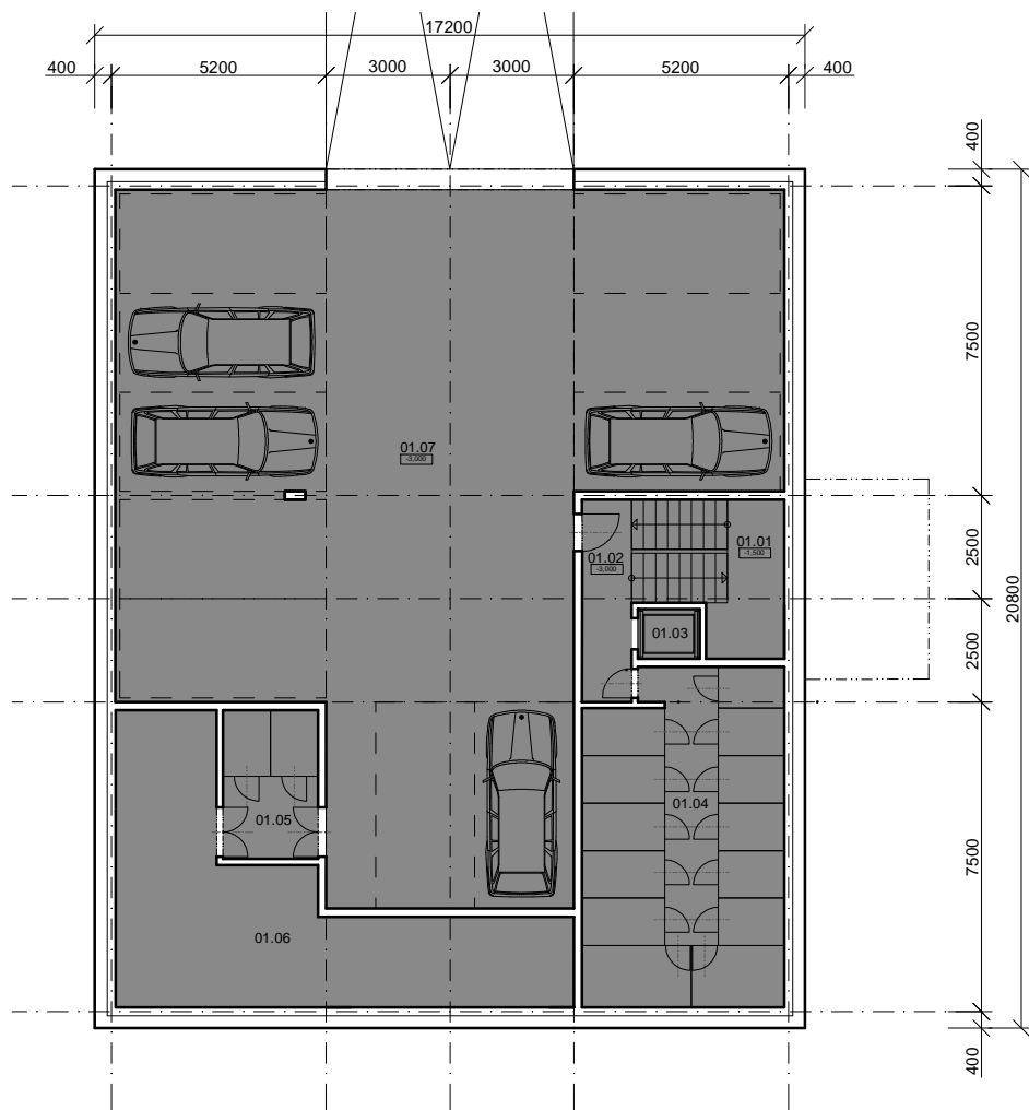
PÔDORYS 1.PP
