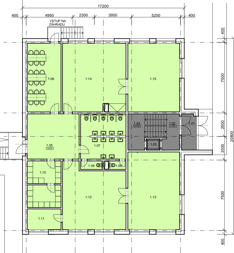
PÔDORYS 1.NP - BD TYP 3 - MATERSKÁ ŠKÓLKA
