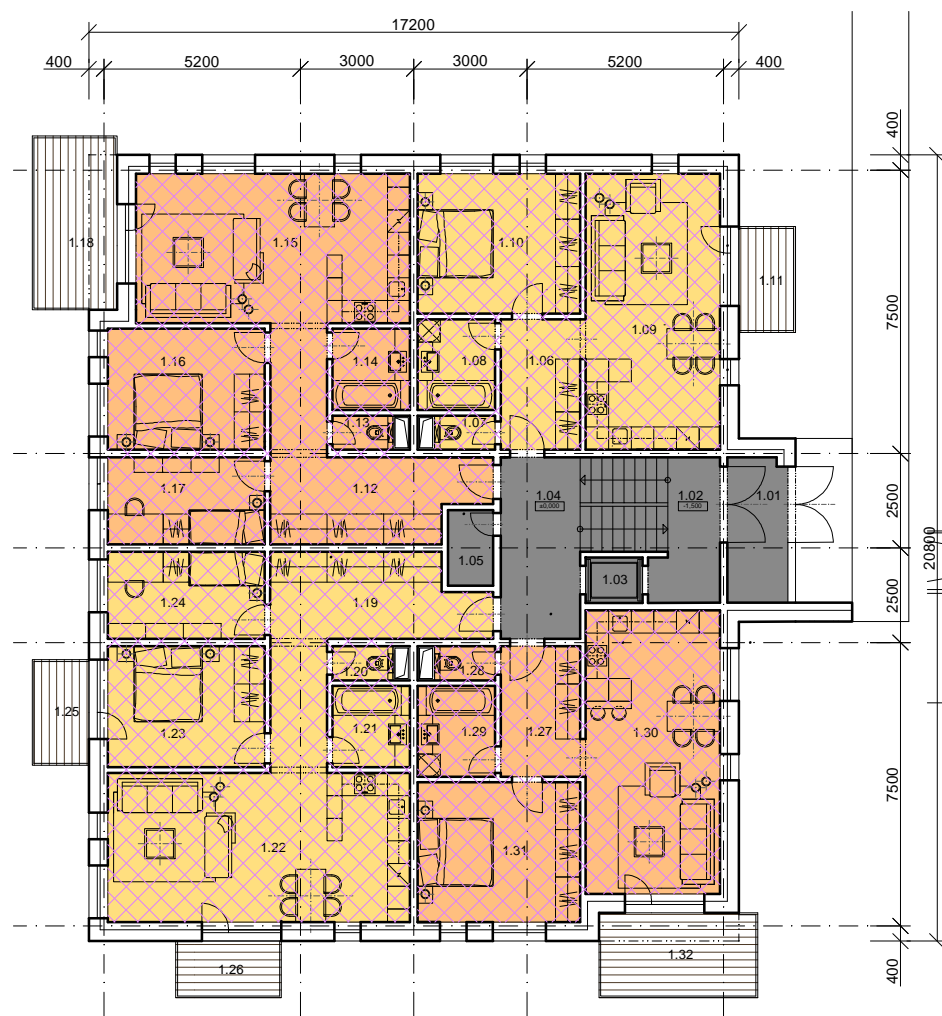
PÔDORYS 1.NP - BD TYP 2
