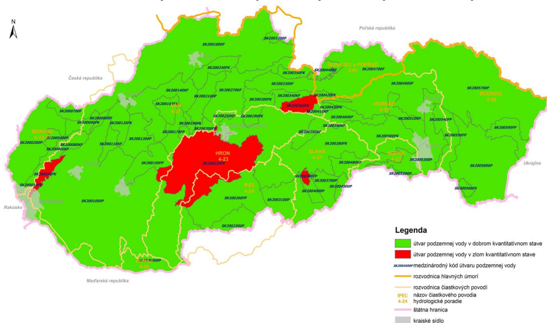
Obrázok 6: Kvantitatívny stav útvarov podzemných vôd v predkvartérnych horninách
