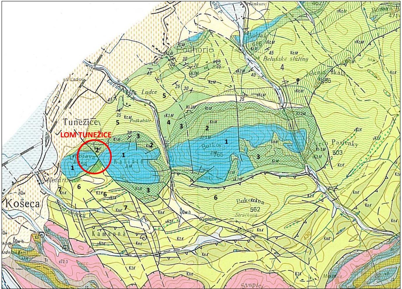
Výsek z geologickej mapy Strážovských vrchov (M. Mahel, 1981)
