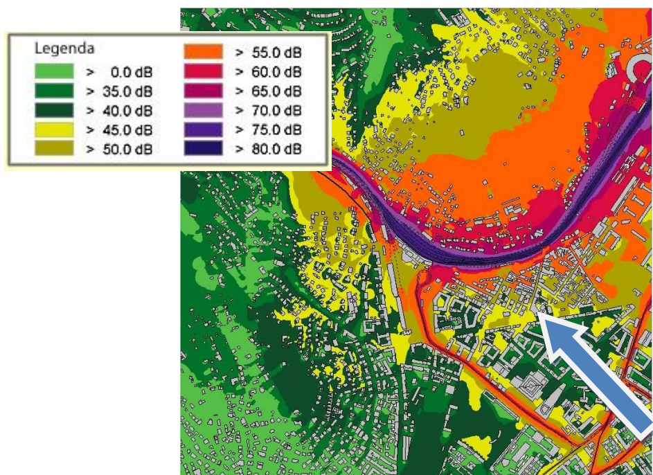
Obr. 4 plošná mapa hladiny L noc pre železničnú dopravu :
