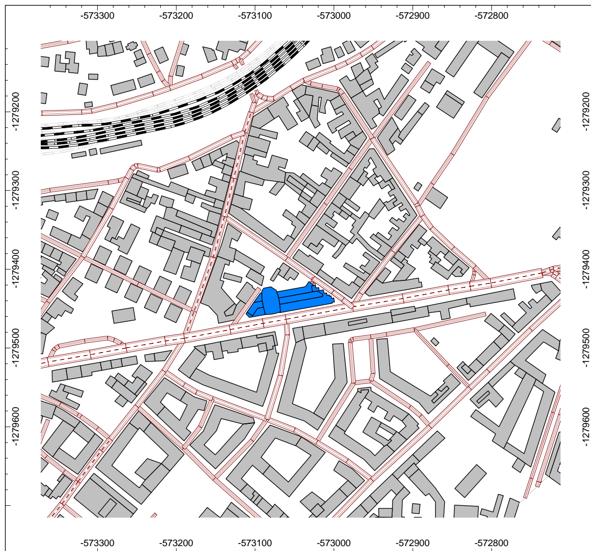
Obr. 7 výpočtový model s posudzovaným objektom
