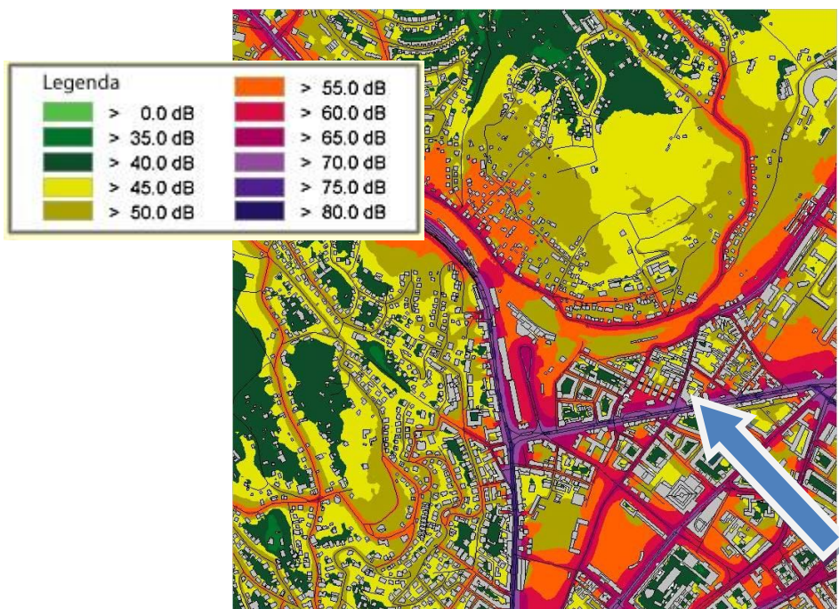
Obr. 3 plošná mapa hladiny L noc pre automobilovú dopravu :
